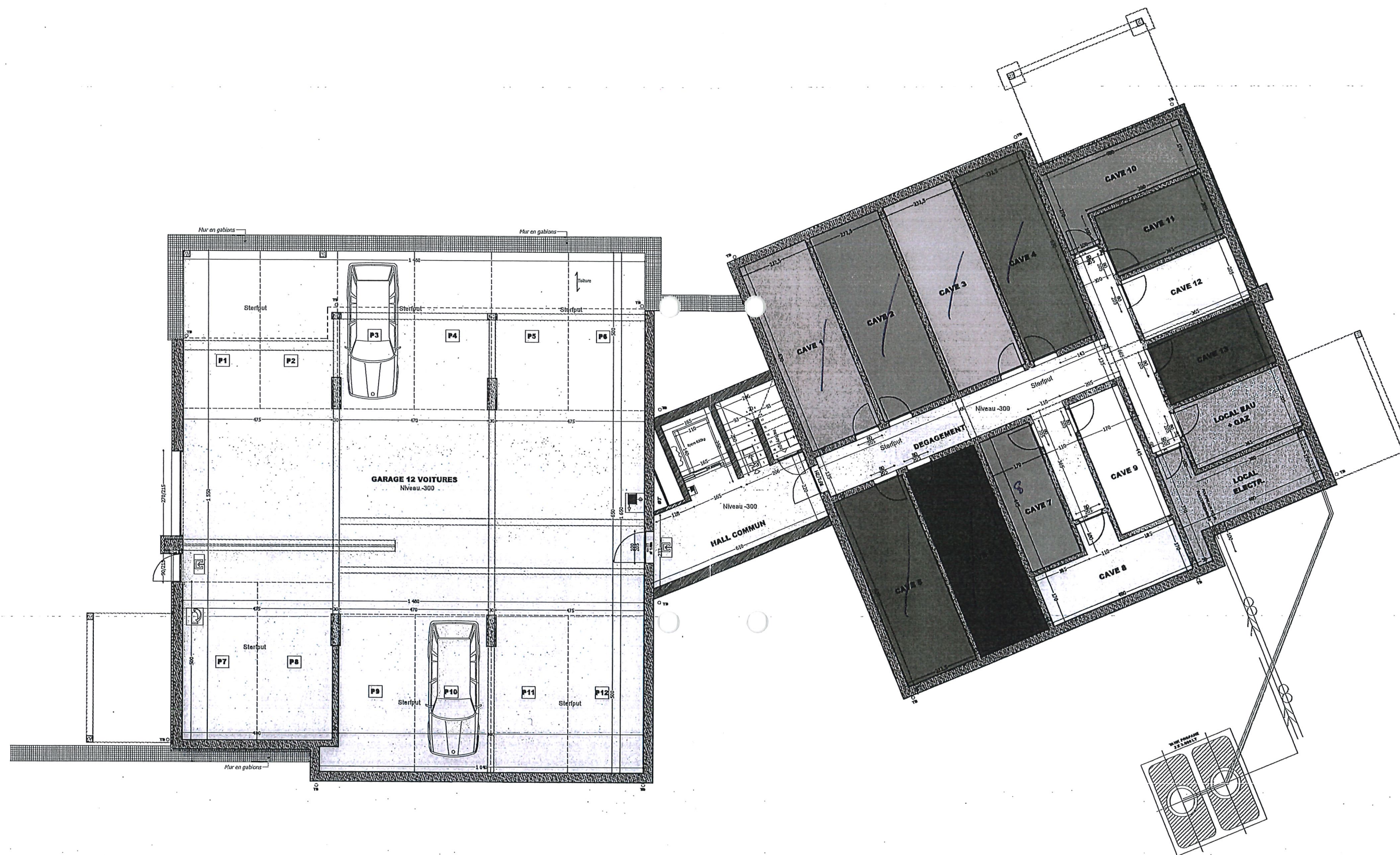
VUE EN PLAN - GARAGES et CAVES - A3 - 1/120
