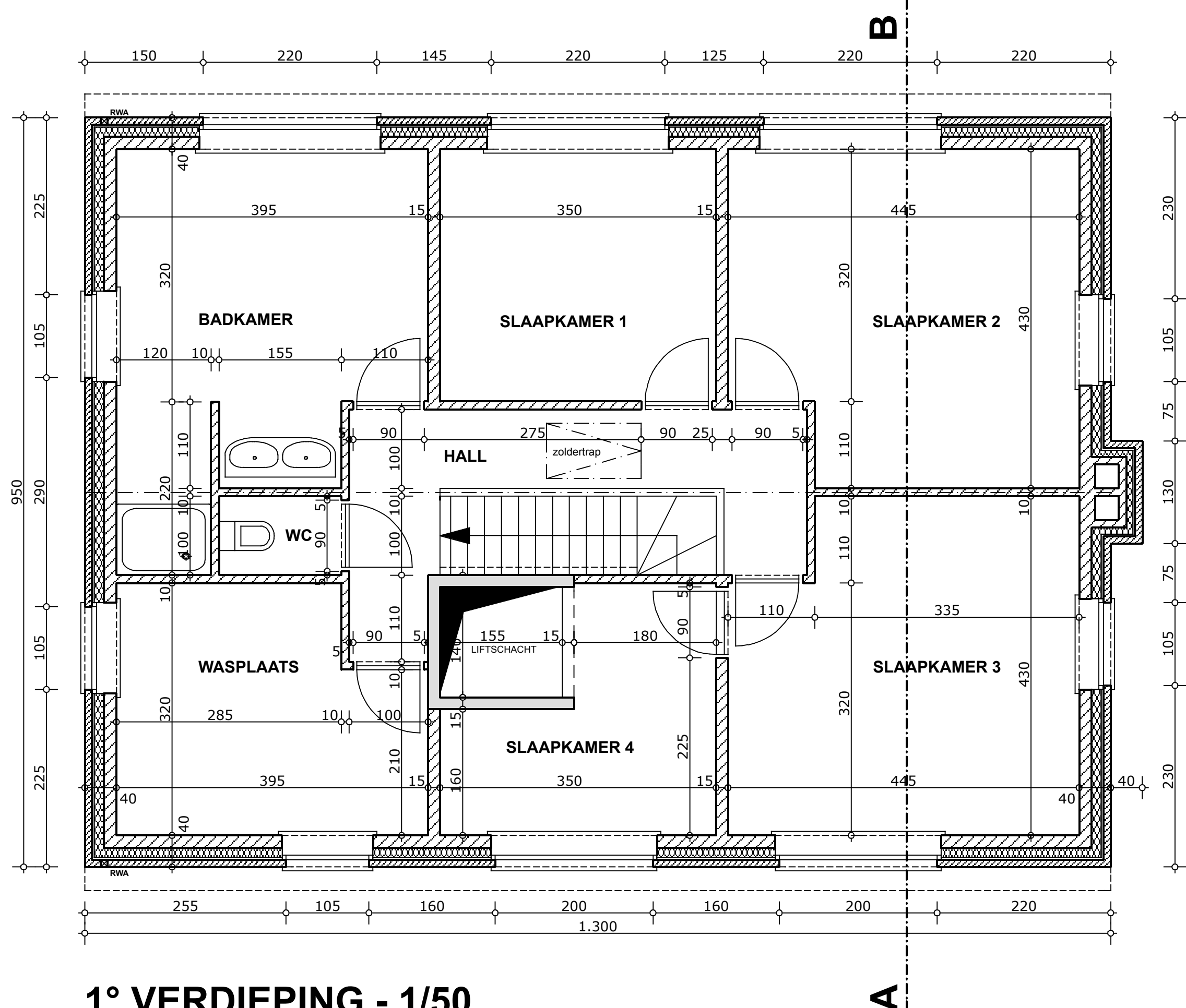
1° VERDIEPING - 1/50
