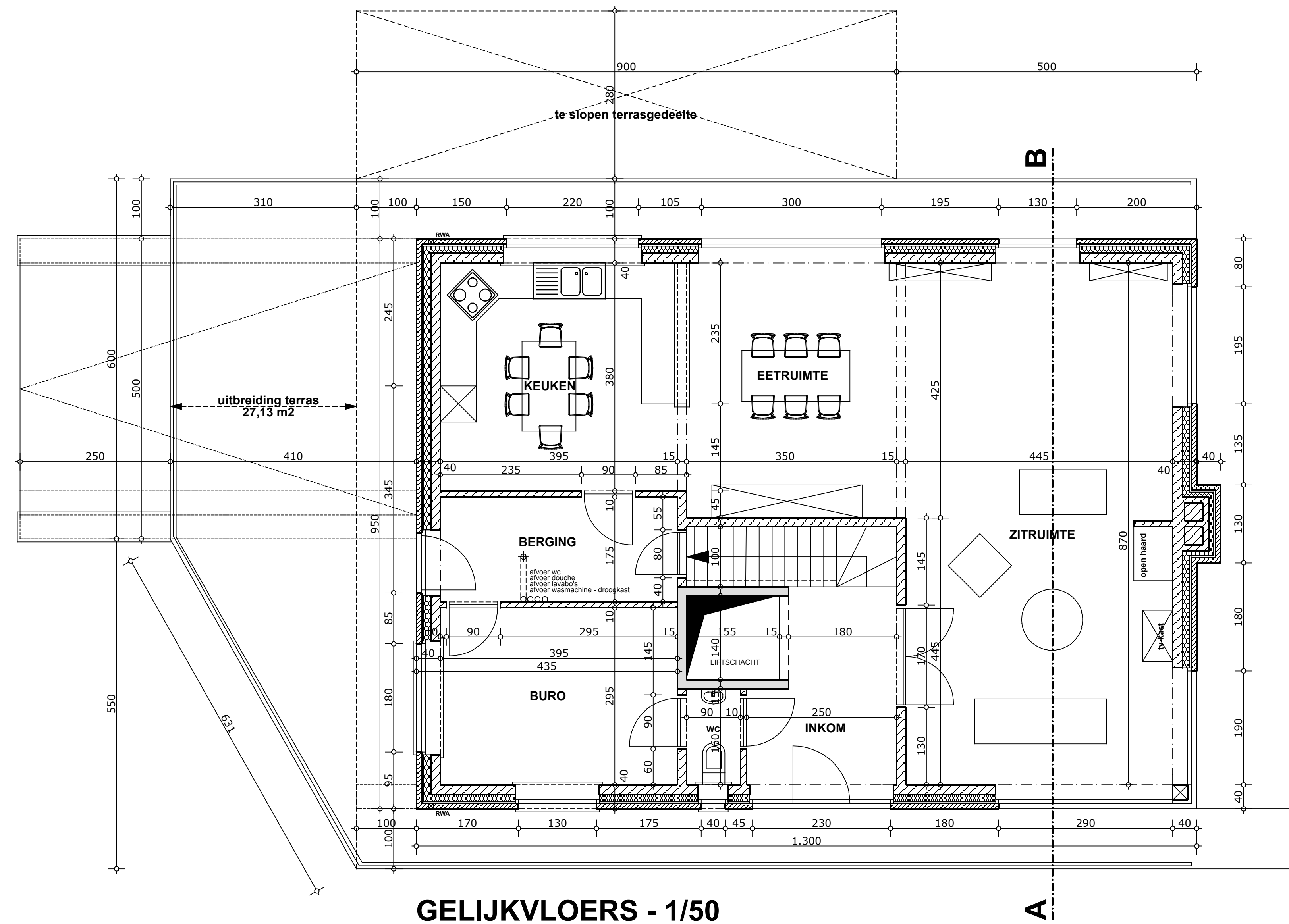
GELIJKVLOERS - 1/50
