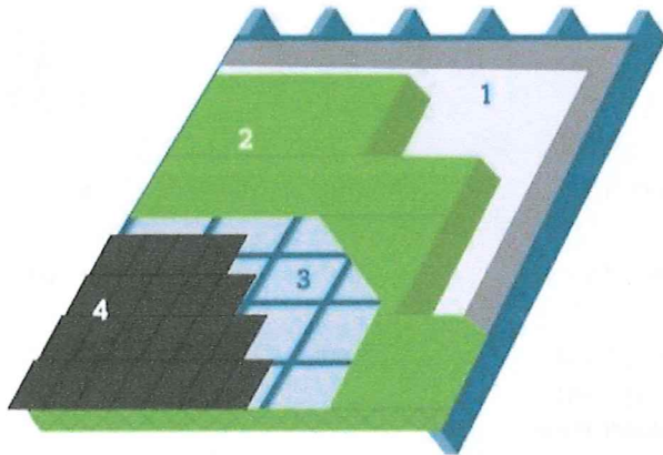
1. Dampfscherm | 2. Isolatatie | 3. Onderdak | 4. Dakbekleding
