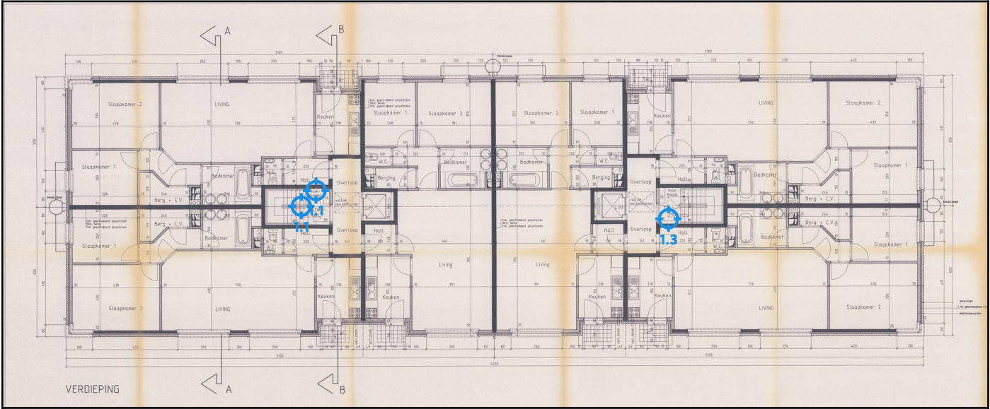
Legende van plan 1.6: Verdieping 5
