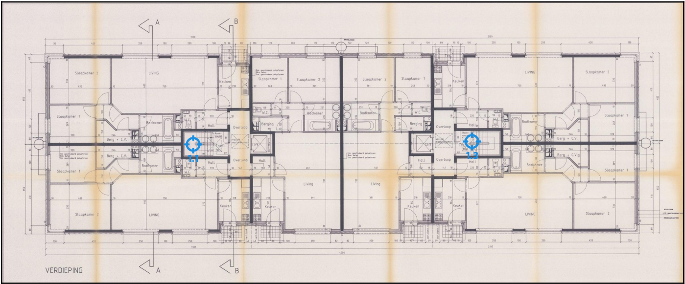
Legende van plan 1.5: Verdieping 4
