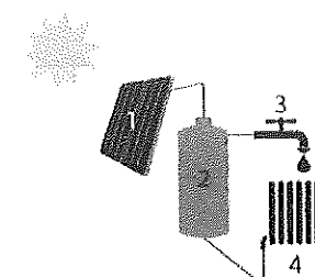
1 Zonnecollector | 2 Opslagvat zonneboiler | 3 Sanitair warm water | 4 Aan de slinger voor ruimteverwarming (radiator)
