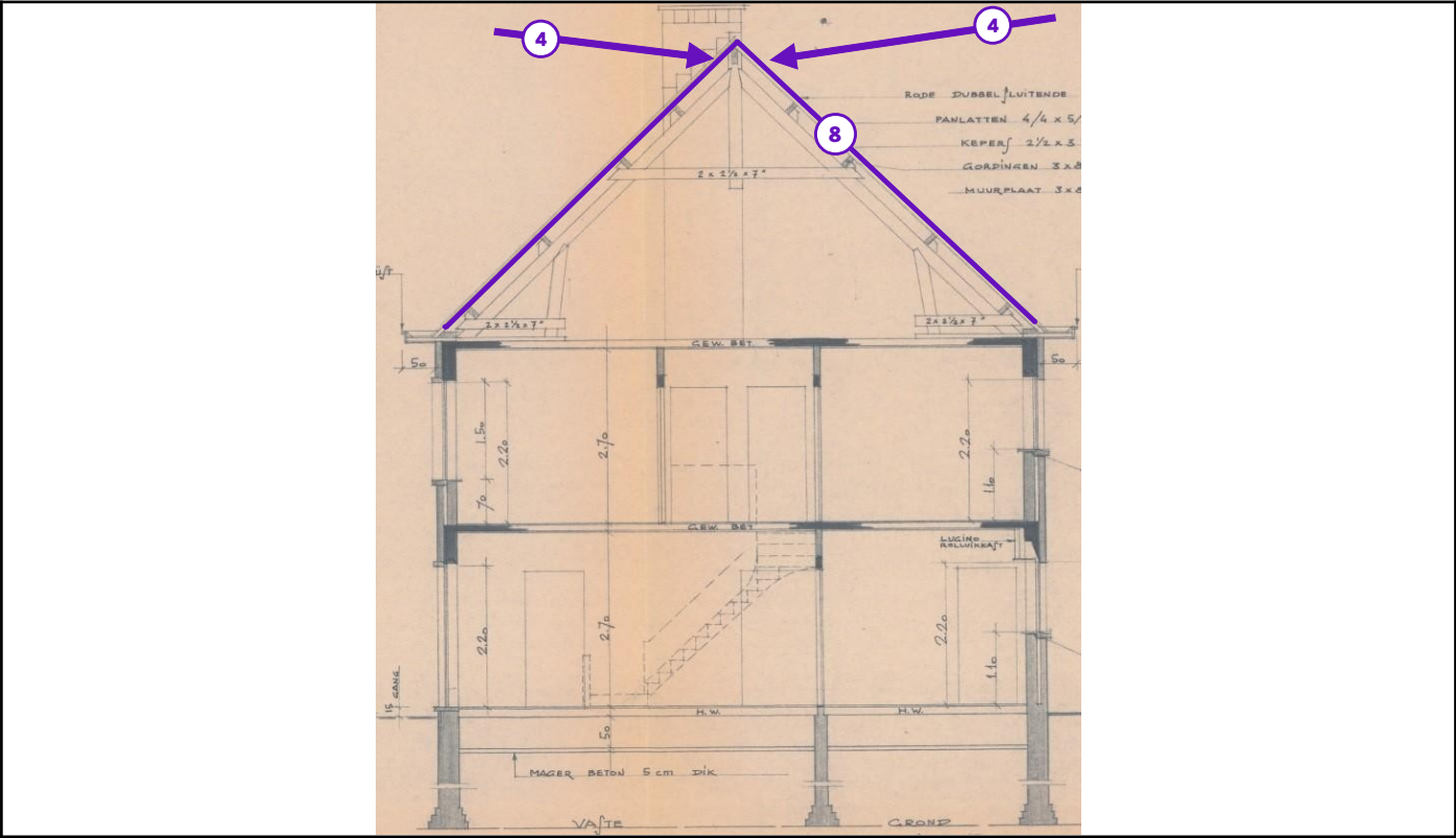
Legende van plan 1.7: doorsnede: onderdak-schouwen
