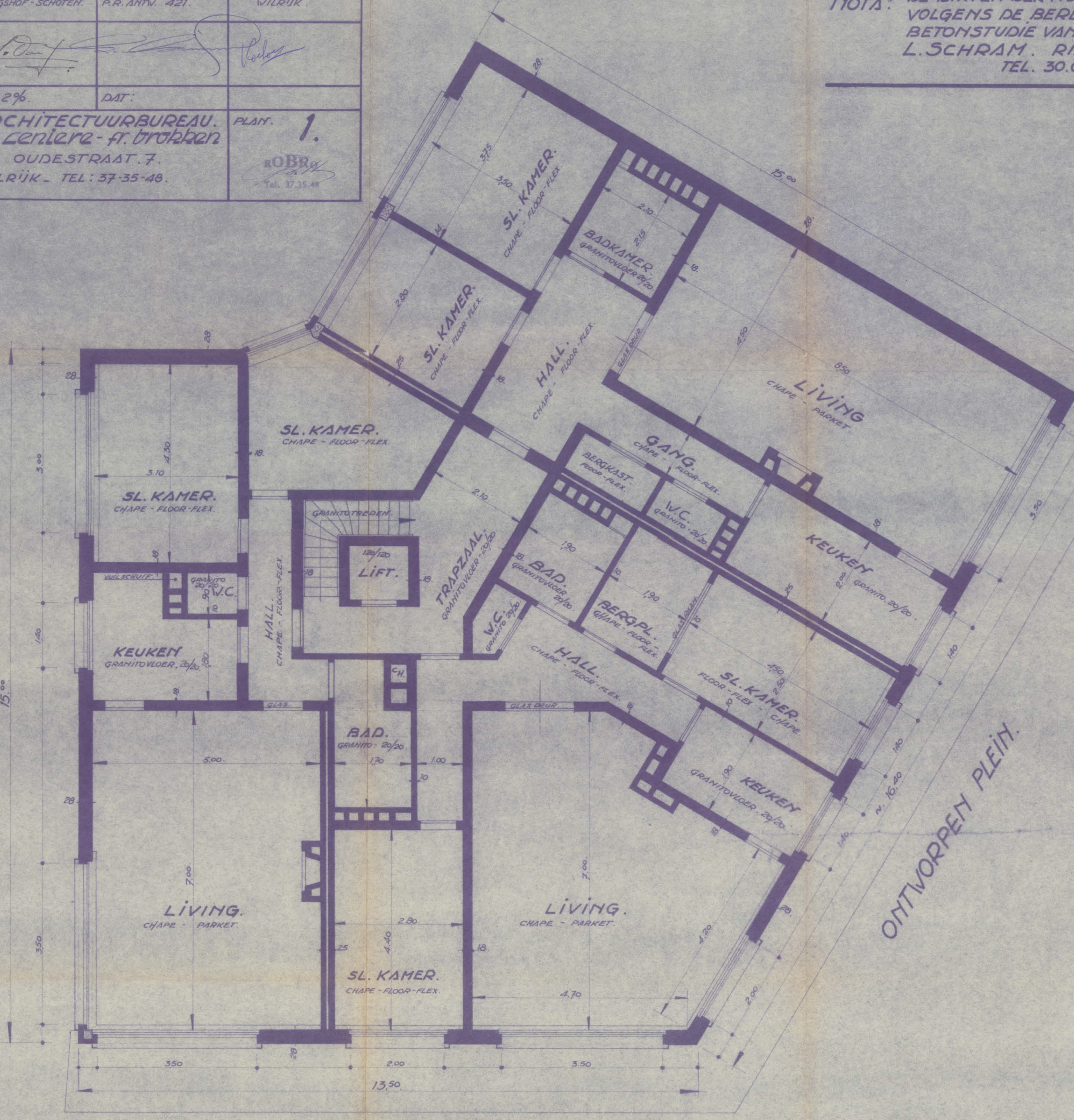
1: 2: 3: 4: VERDIEPING. GROENENBORGERLAAN.
