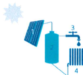
1. Zonnecollector | 2. Opslagvat zonneboiler | 3. Sanitair warm water | 4. Afgift-element voor ruimteverwarming (optioneel)
