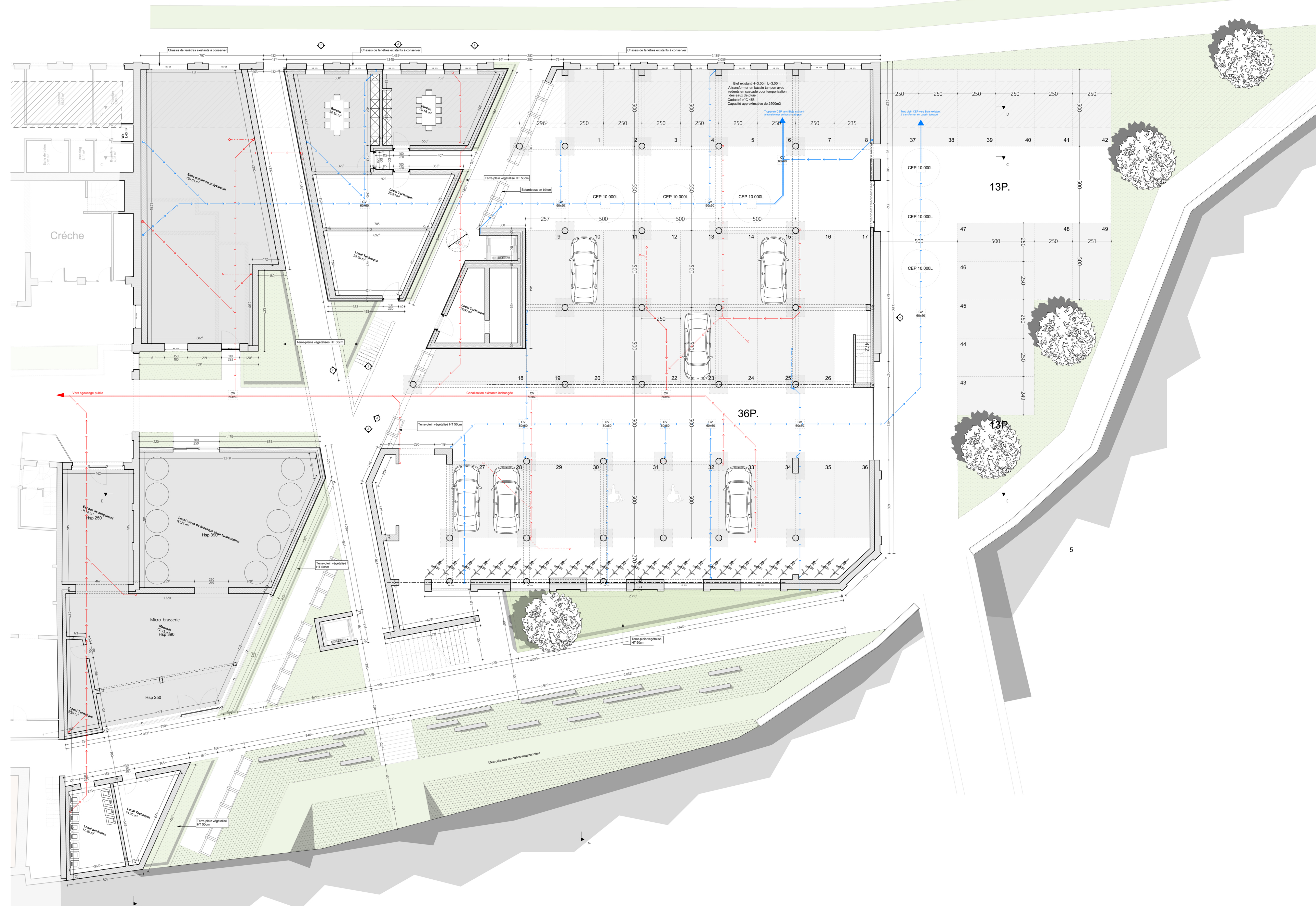
Rez-de-chaussée 1/100
