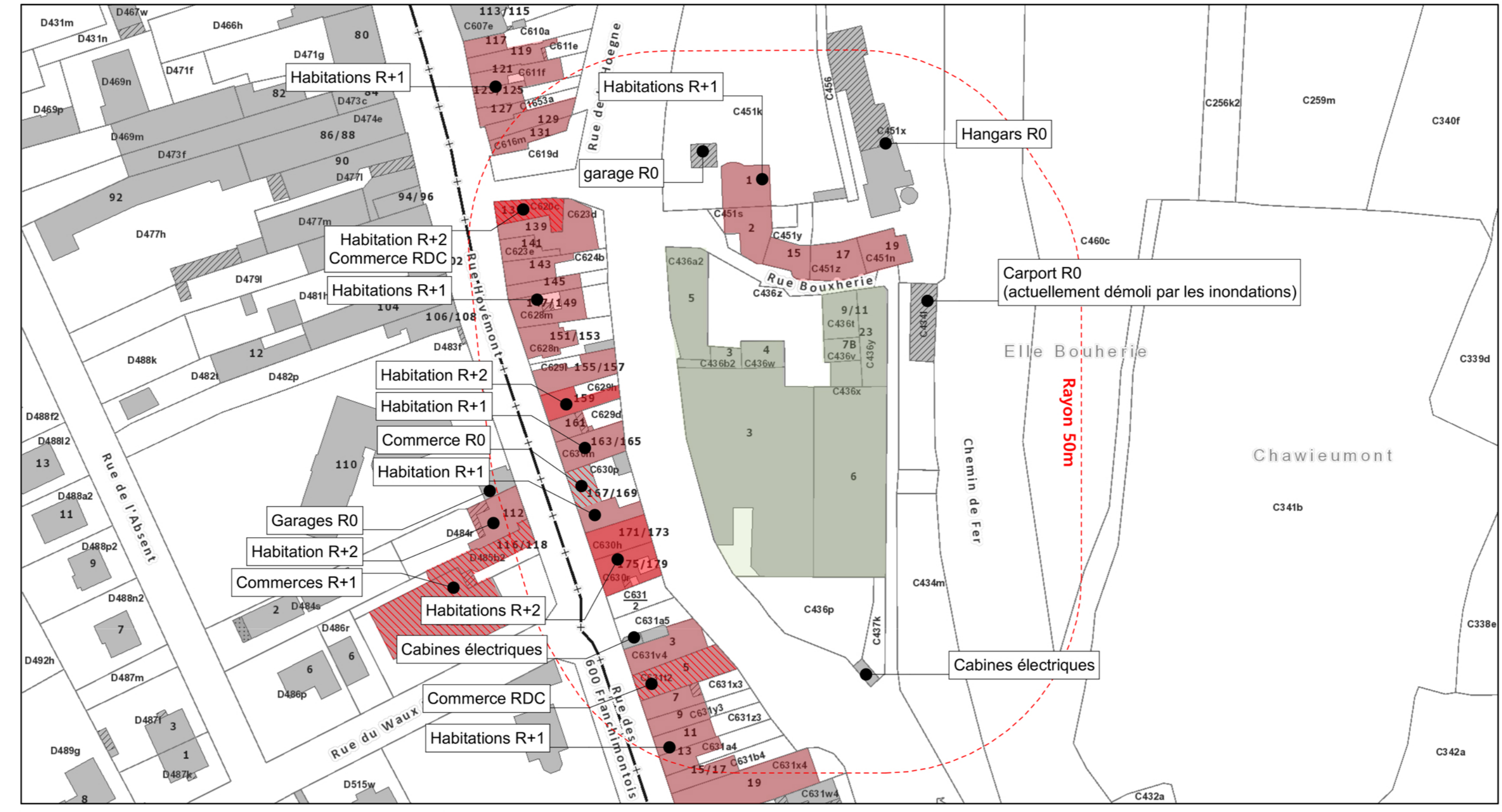
Contexte 1/1000
