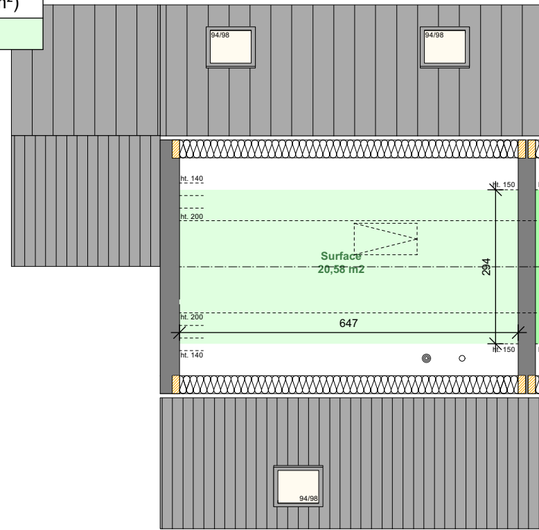
PLAN DES COMBLES
