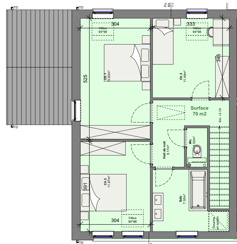
PLAN PREMIER ETAGE
