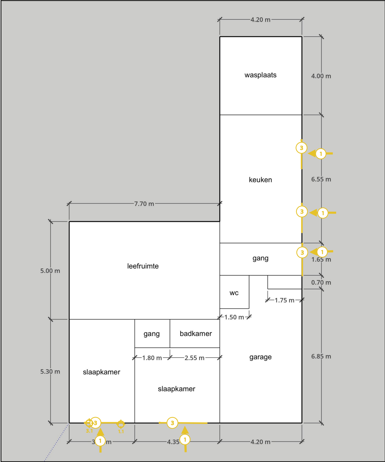
Legende van plan 1.2: Grondplan
