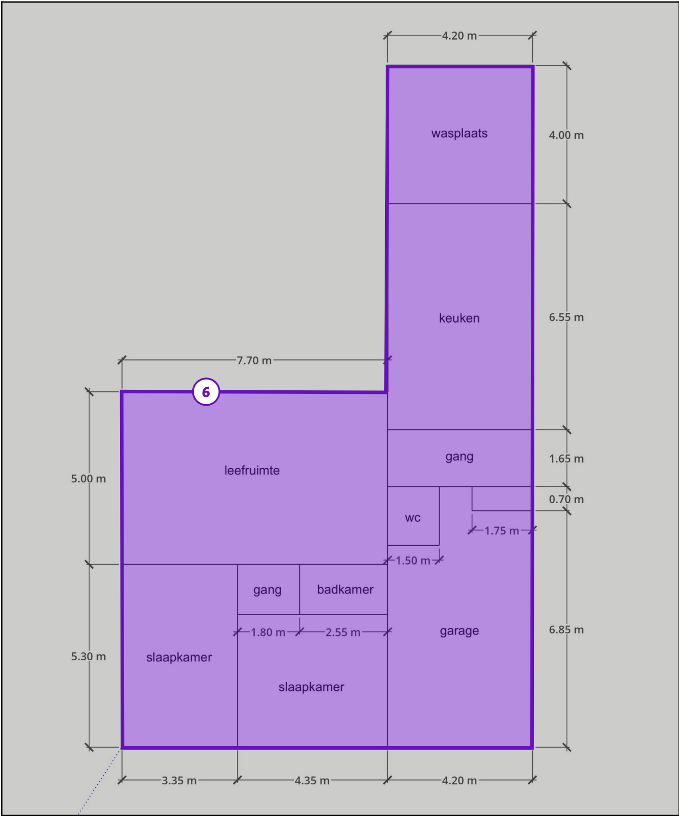
Legende van plan 1.4: Grondplan
