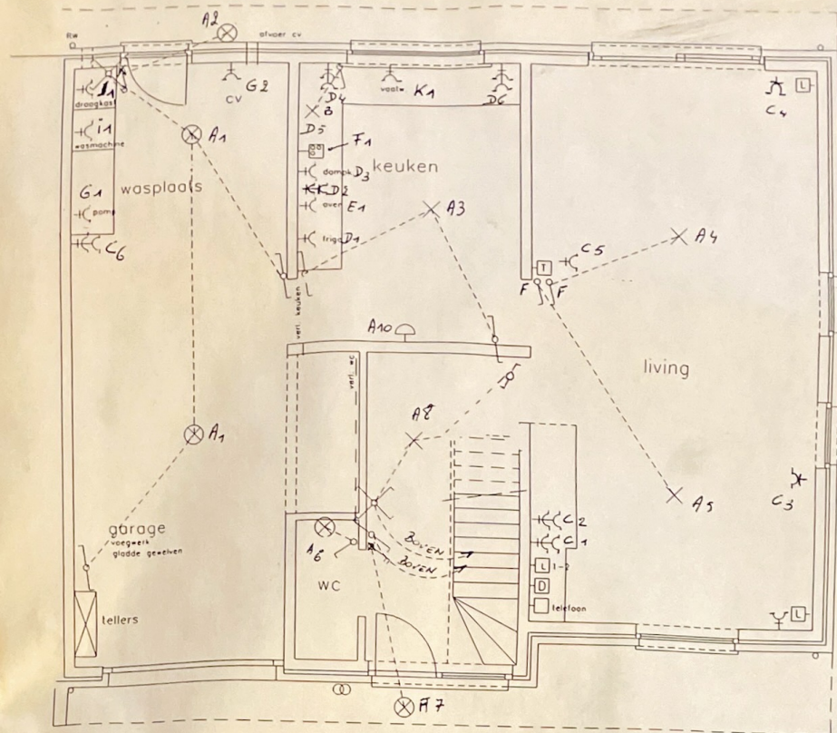
PLAN ELEKTRICITEIT GELIJKVLOERS
