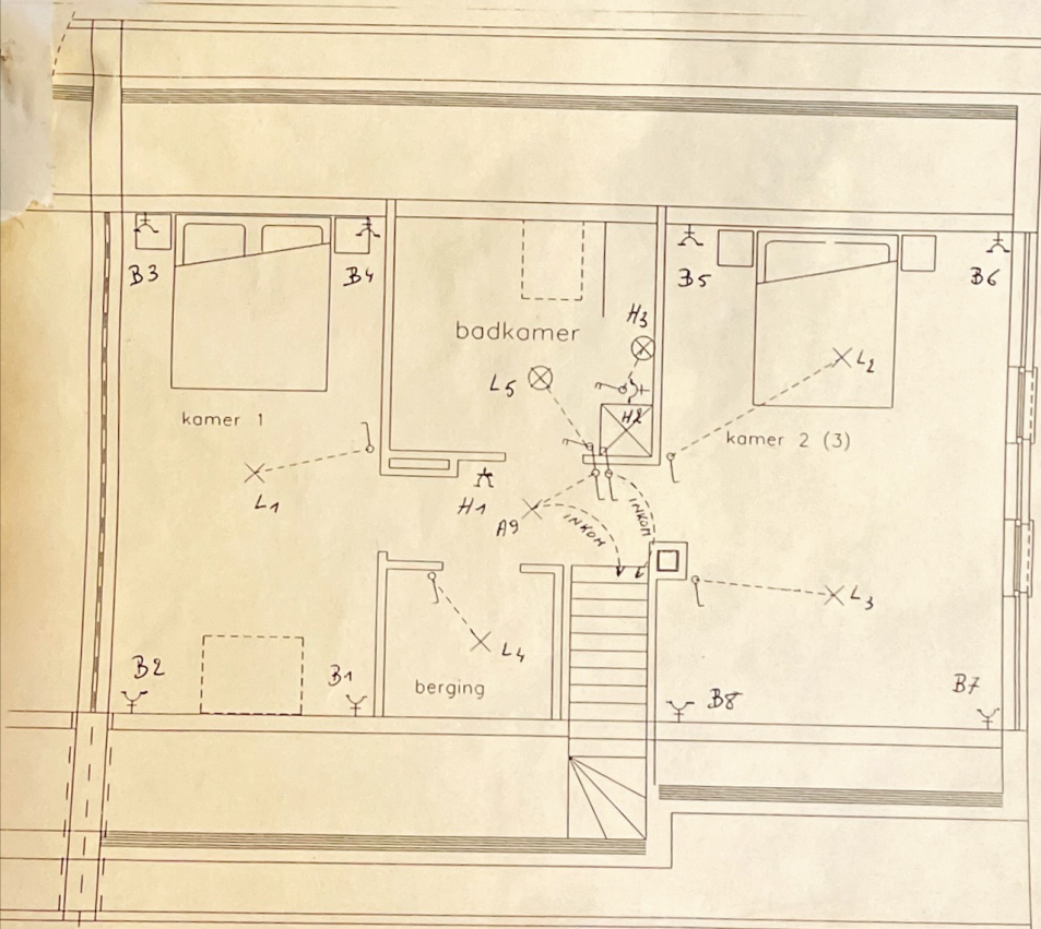
PLAN ELEKTRICITEIT VERDIEPING
