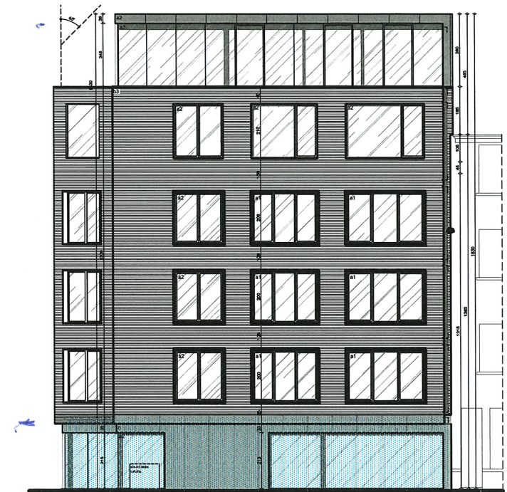
gevel Bordeauxstraat 1/200
