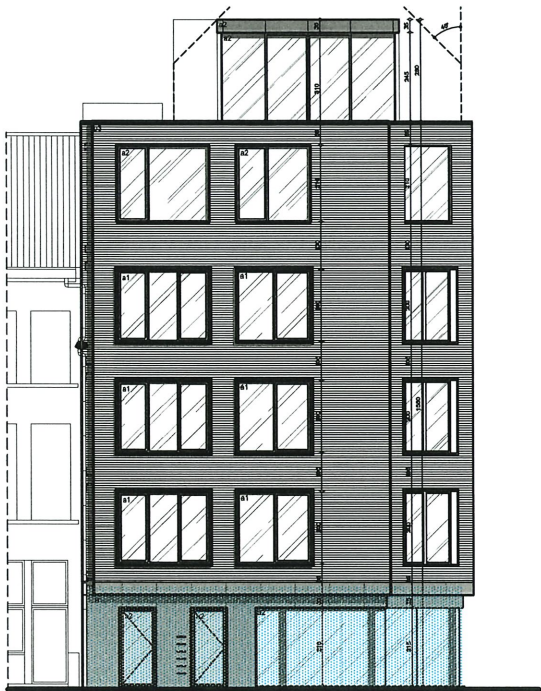
gevel Londenstraat 1/200
