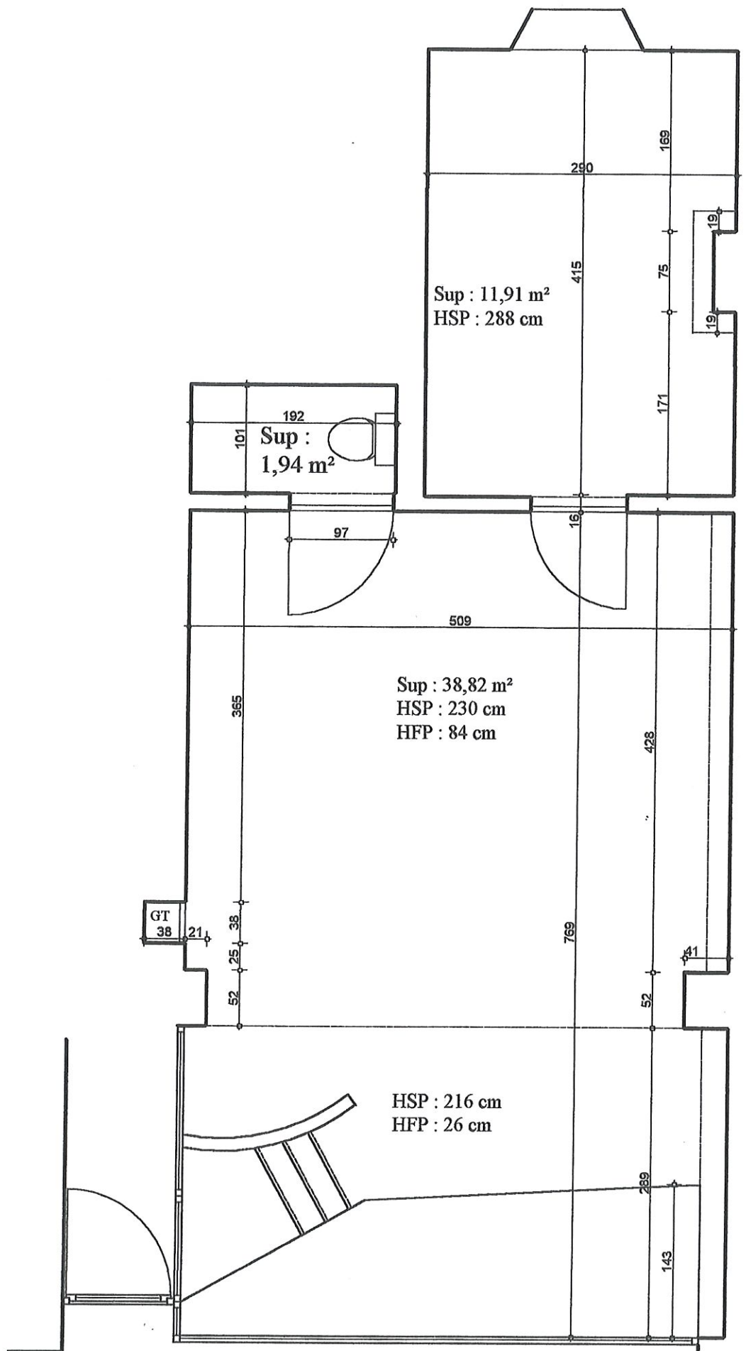
PLAN DU MAGASIN ( Ech : 1/50ème ) sup : 52,67 m 2
