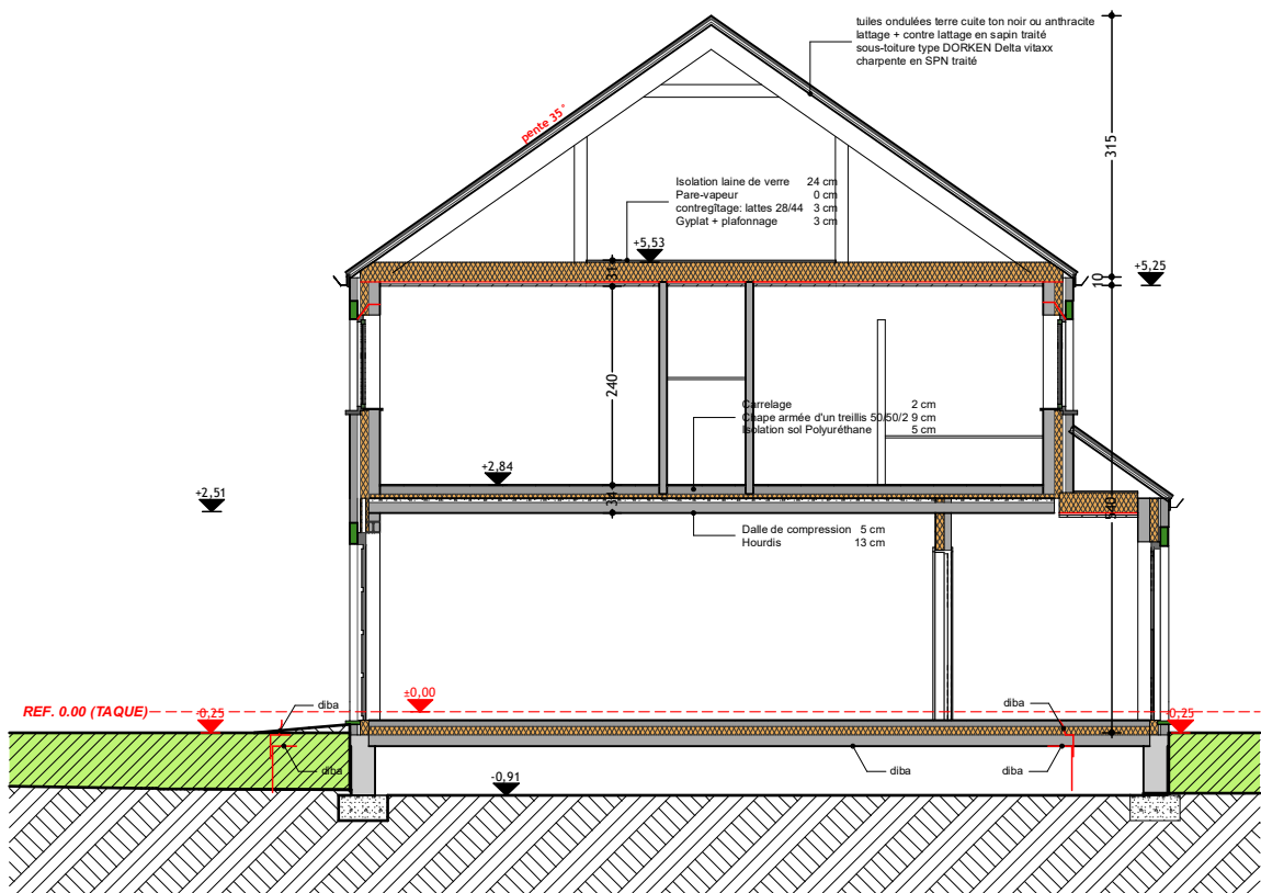
Coupe B6 1:100
