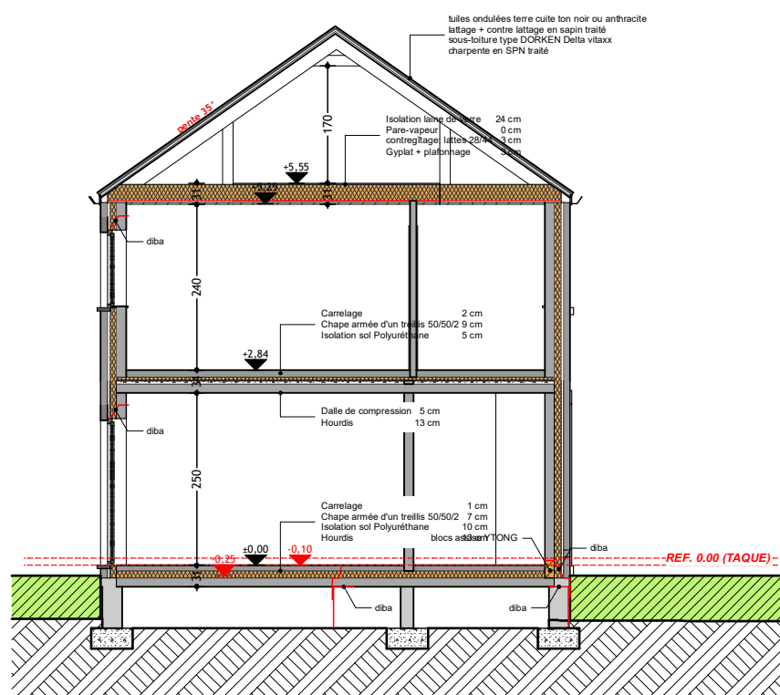
Coupe A5 1:100
