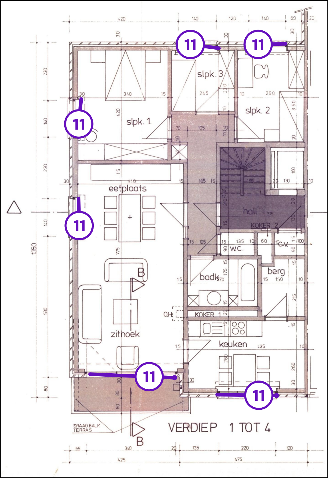
Legende van plan 1.7: Kitwerk tussen raamprofiel en muur
