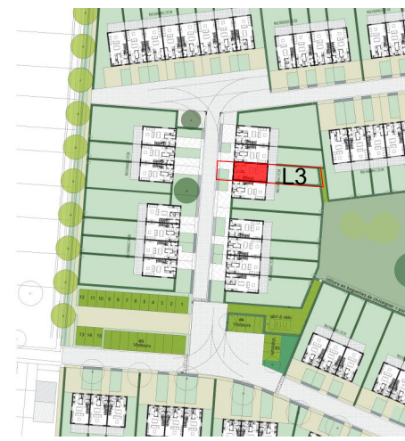
Plan d'implantation
