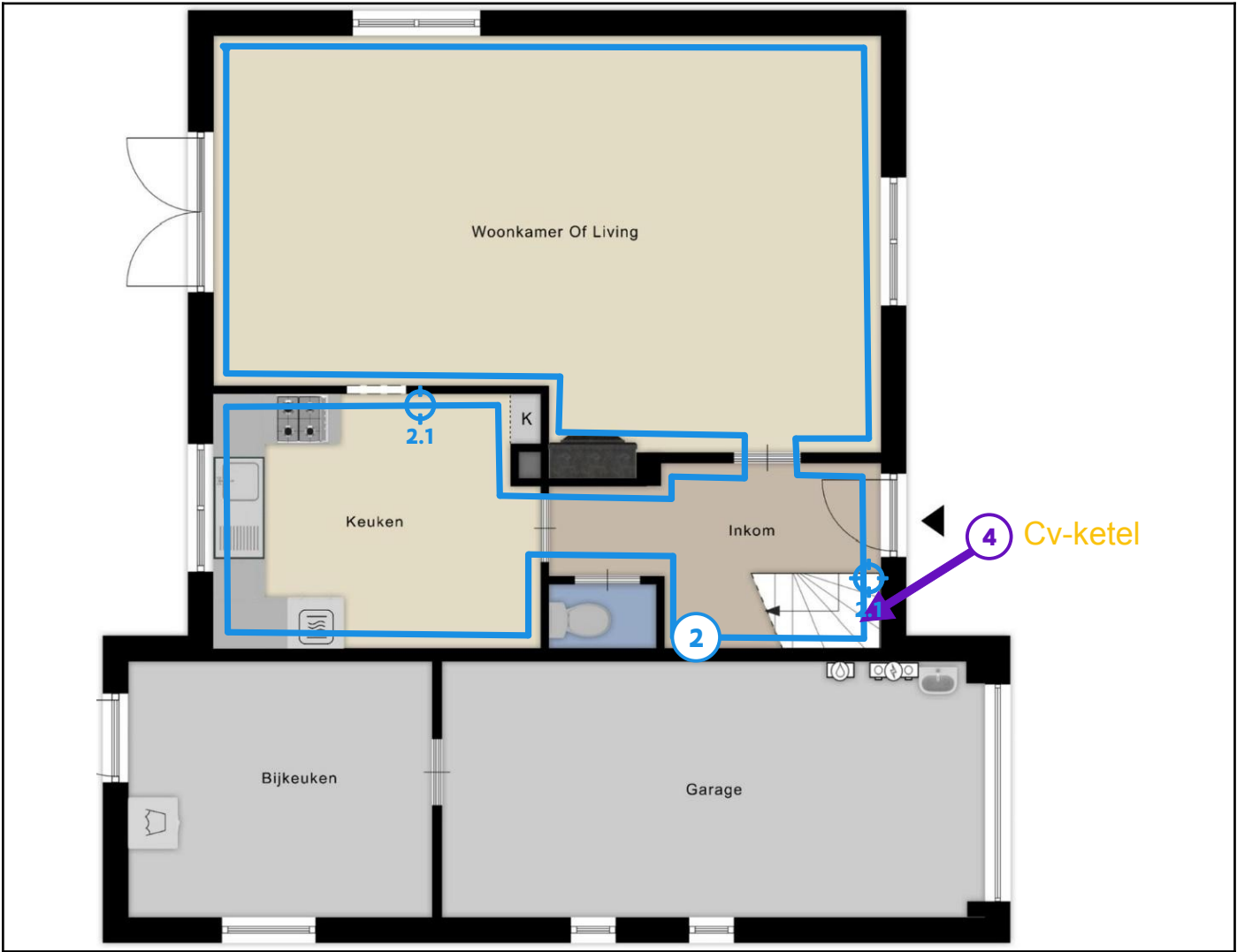
Legende van plan 1.2: Plan gelijkvloers (1)
