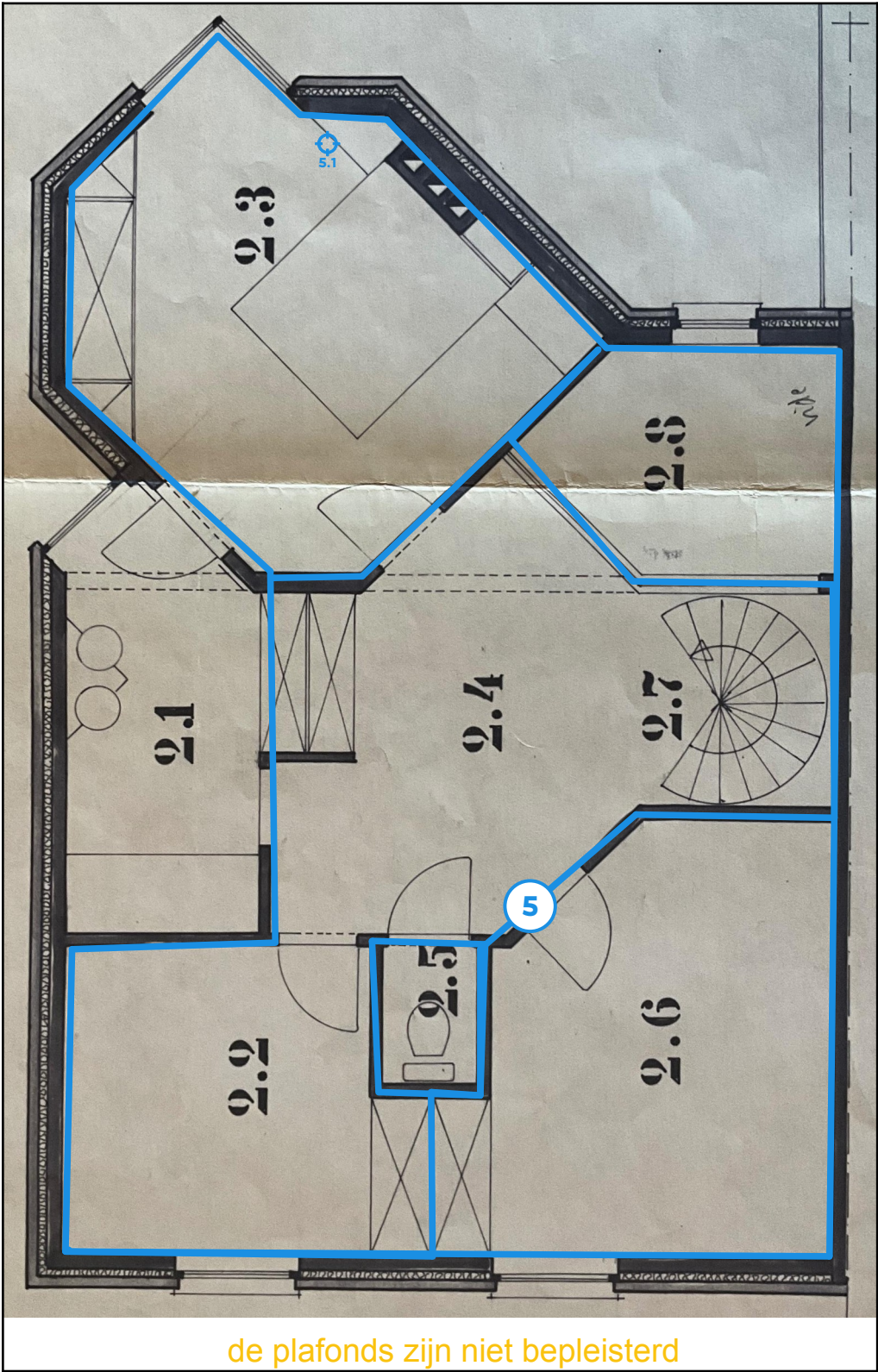
Legende van plan 1.3: 2de verdiep
