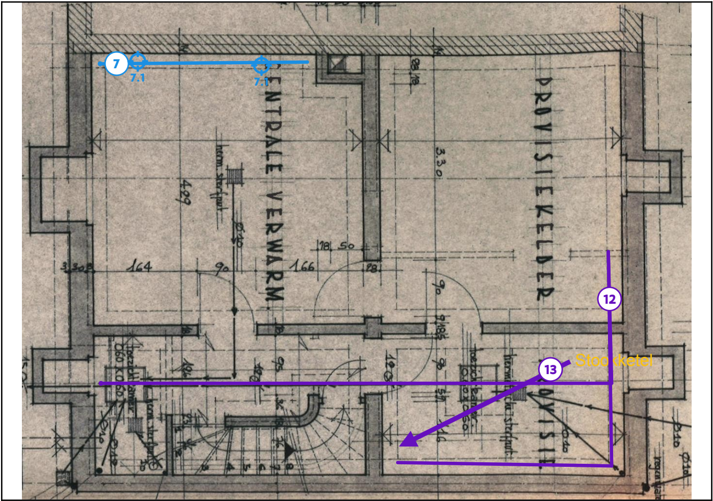
Legende van plan 1.2: Plan kelder
