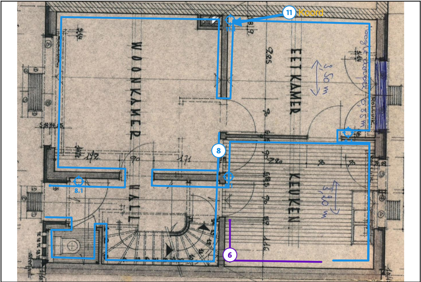
Legende van plan 1.3: Plan gelijkvloers (1)
