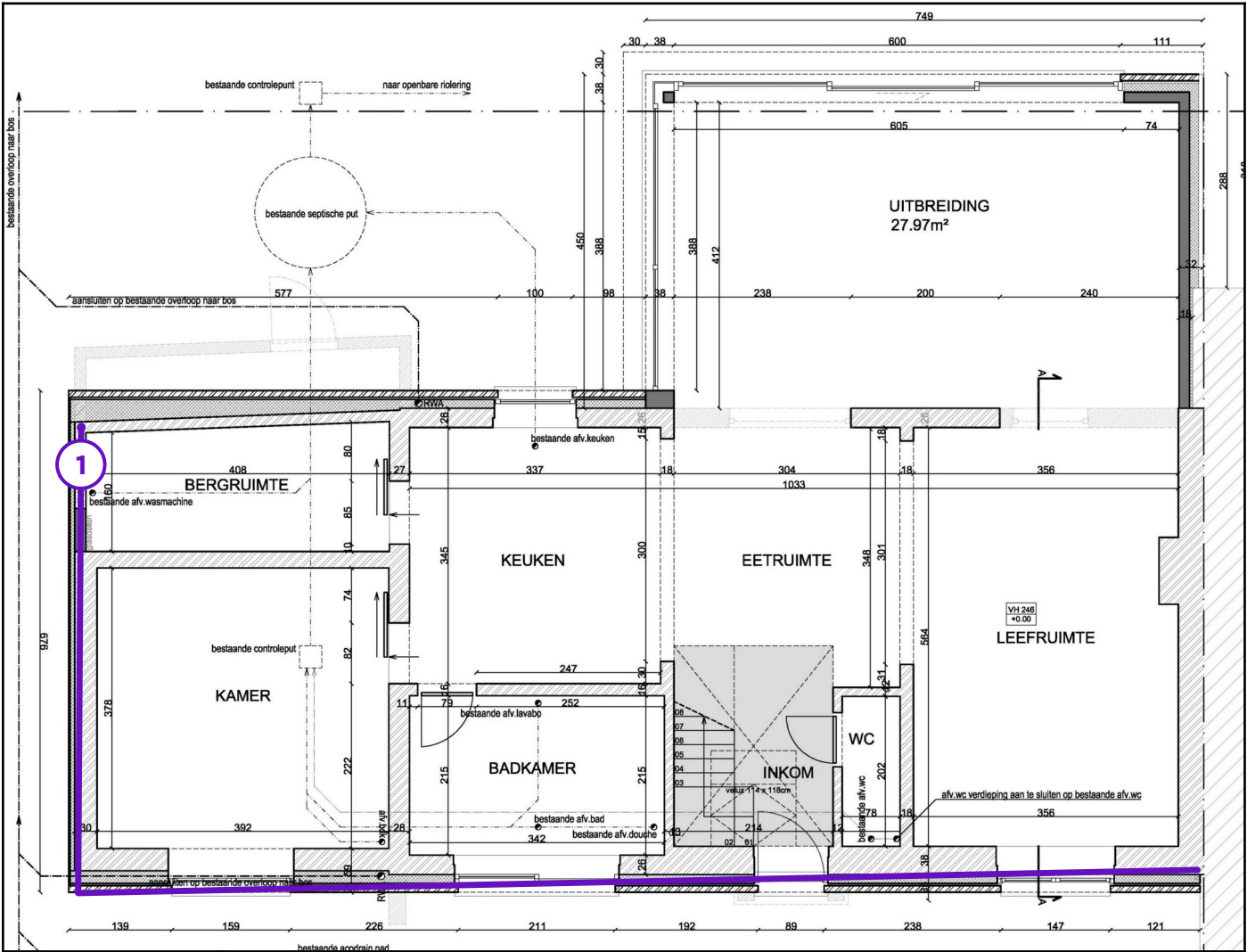
Legende van plan 1.2: Gelijkvloers plan
