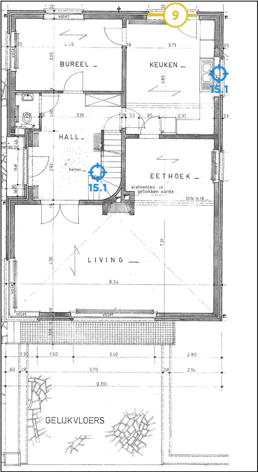
Legende van plan 1.4: Plan gelijkvloers (1)
