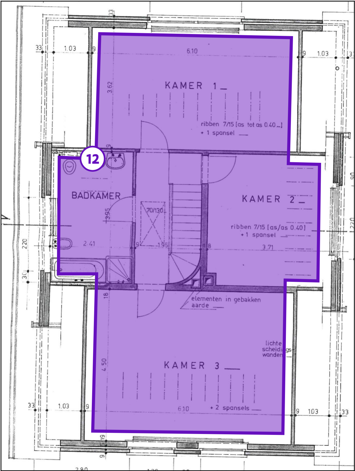
Legende van plan 1.6: Plan 1e verdiep
