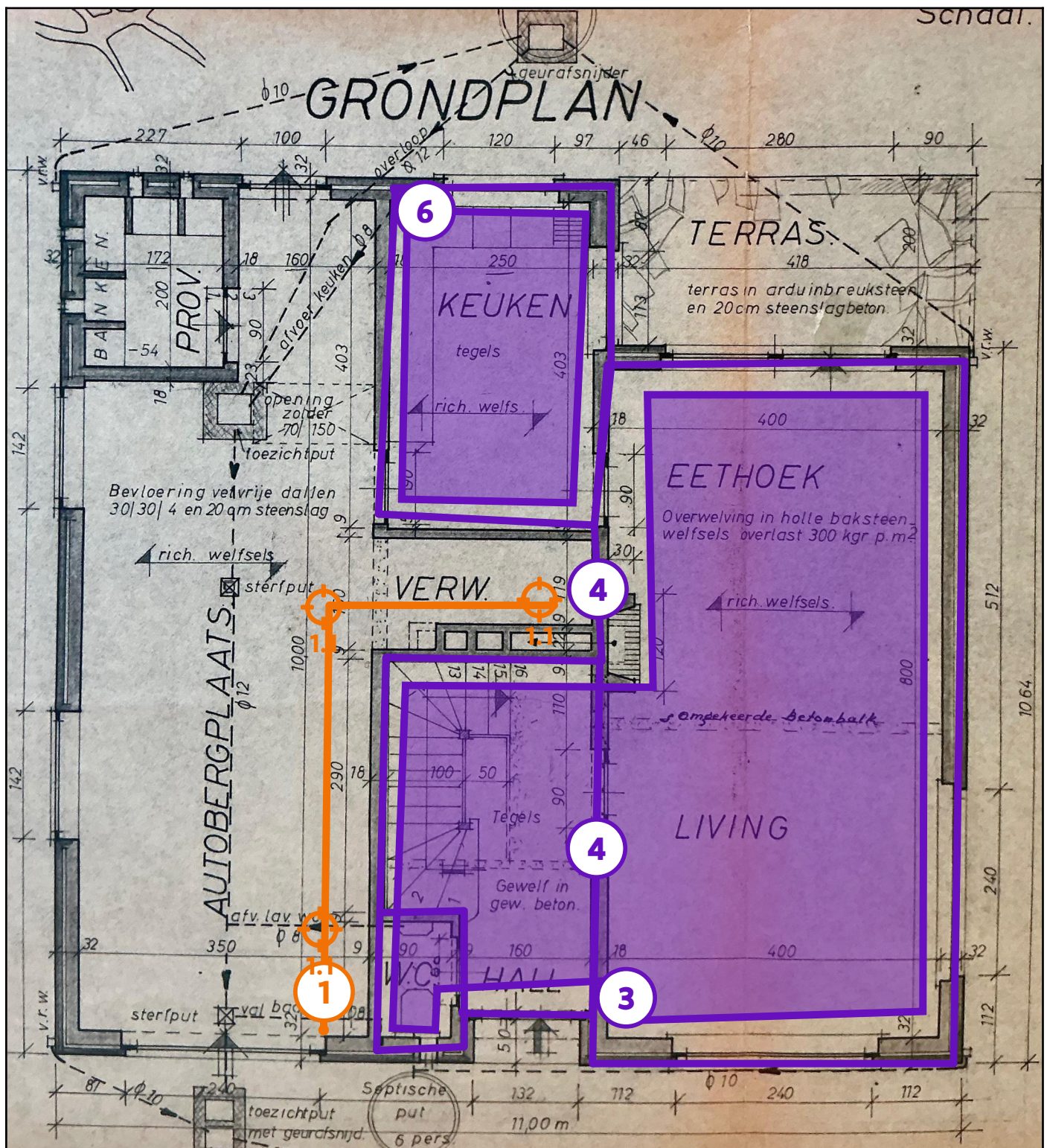
Legende van plan 1.4: Gelijkvloers plan
