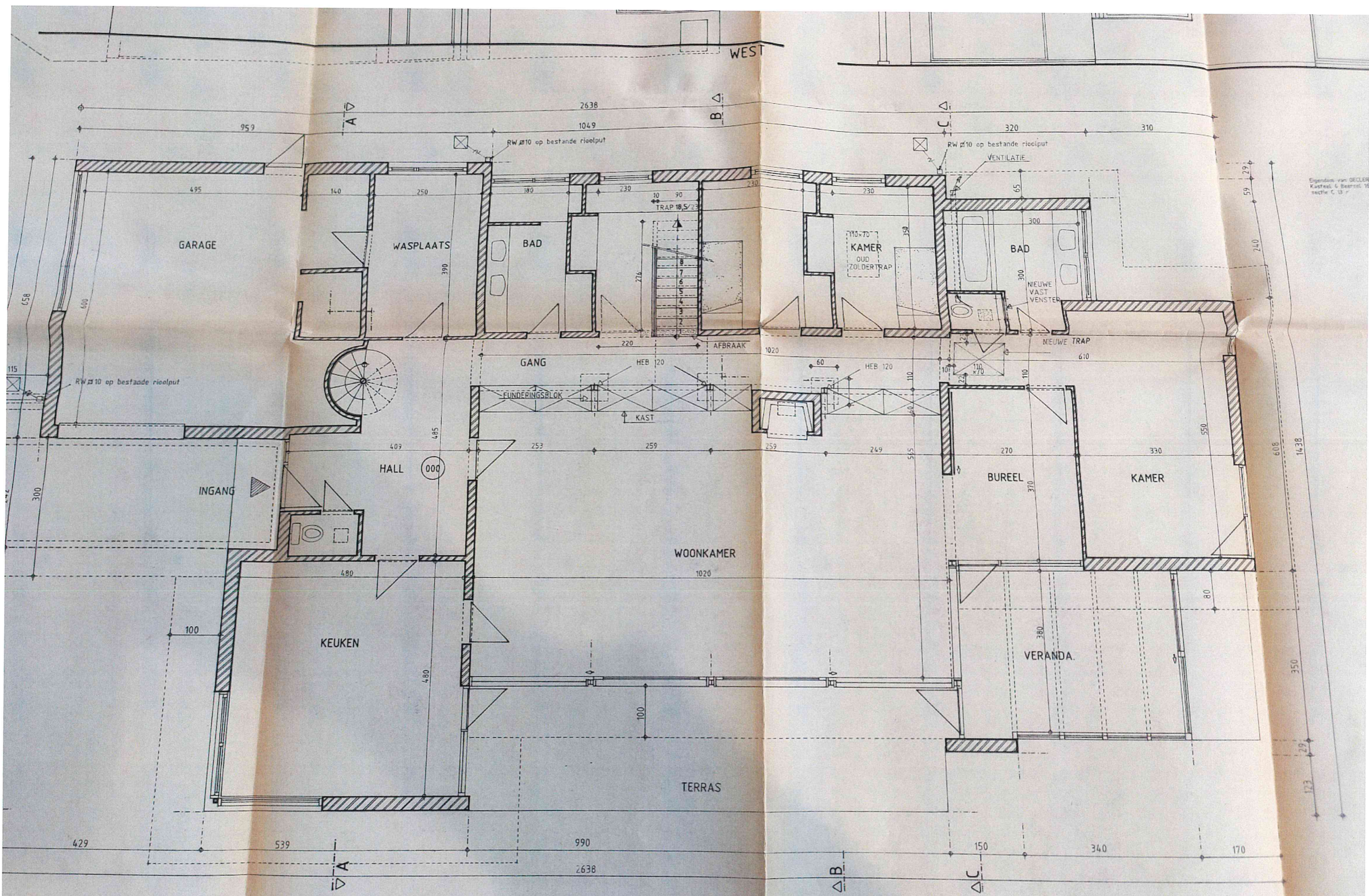
GELIJKVLOERSPLAN
