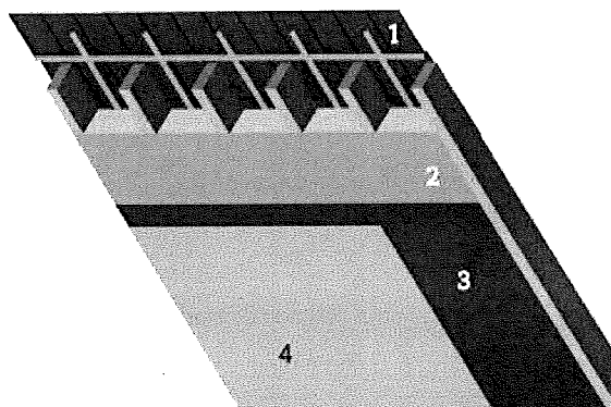
1. Onderdak | 2. Isolatie | 3. Dampscreen | 4. binnenafwerking
