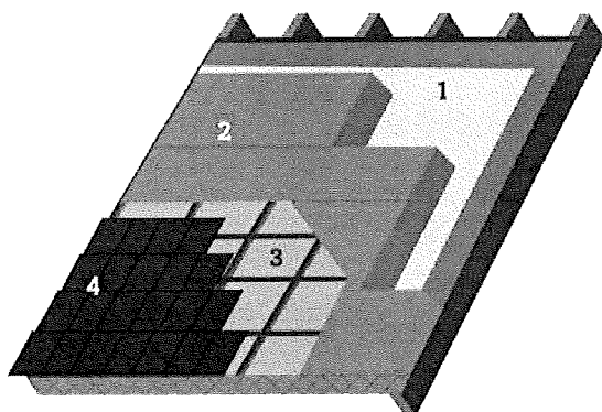
1. Dampscreen | 2. Isolatie | 3. Onderdak | 4. Dakbekleding
