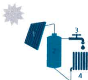
1 Zonnecollector 2 Opslagvat zonneboiler 3 Sanitair warm water 4 Afgegeven warmte voor ruimteverwarming (radiator)
