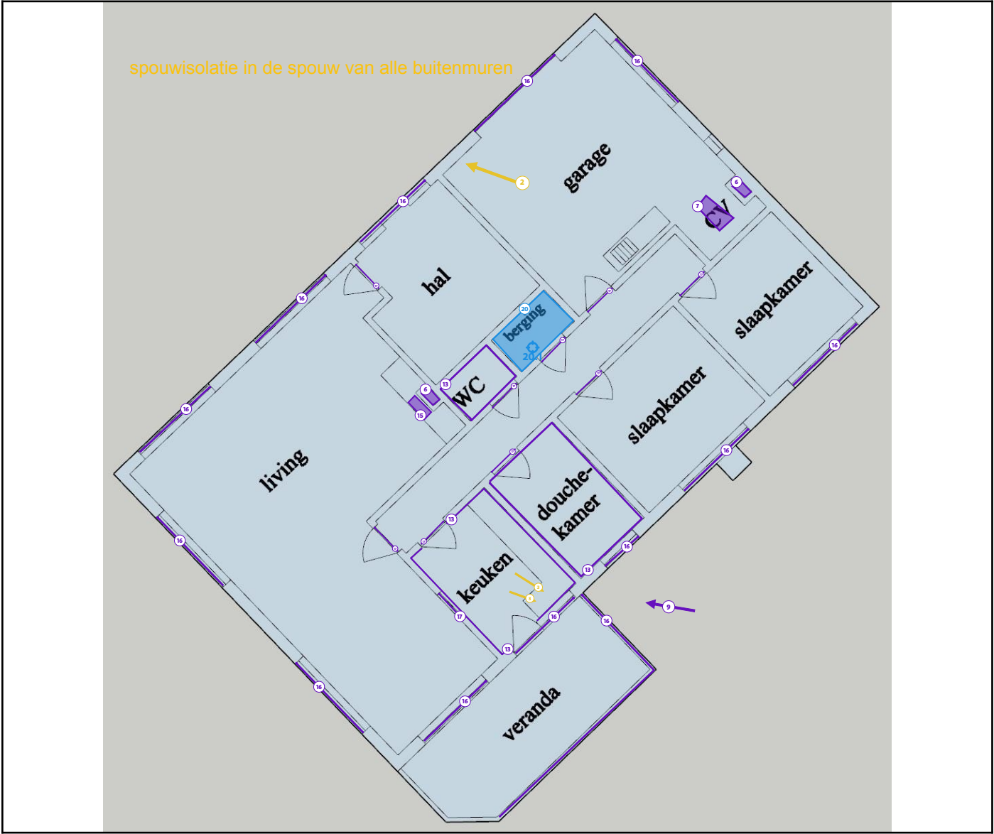
Legende van plan 1.2: grondplan gelijkvloers
