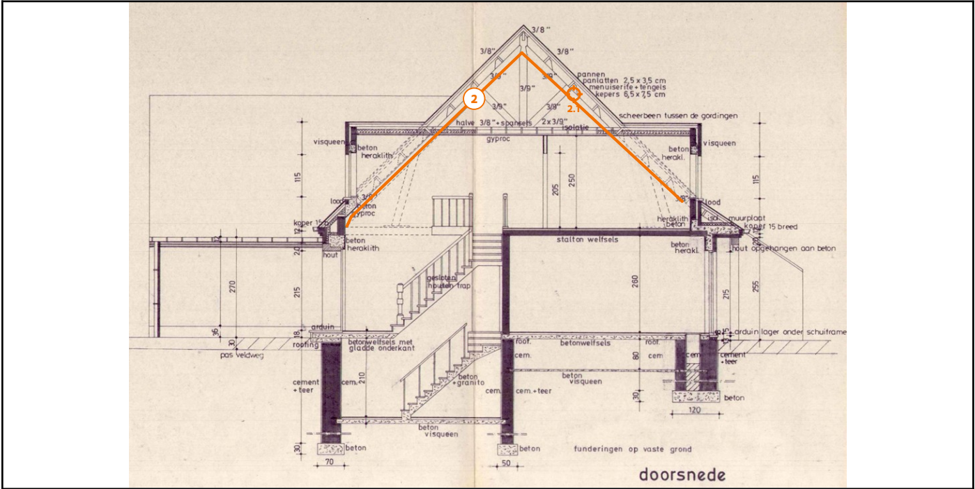
Legende van plan 1.8: Doorsnede
