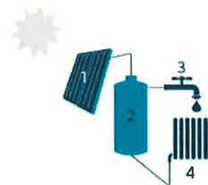
1. Zonnecollector | 2. Opslagvat (boiler) | 3. Sanitair (badkamer) | 4. Verwarmingscircuit (ruimteverwarming)
