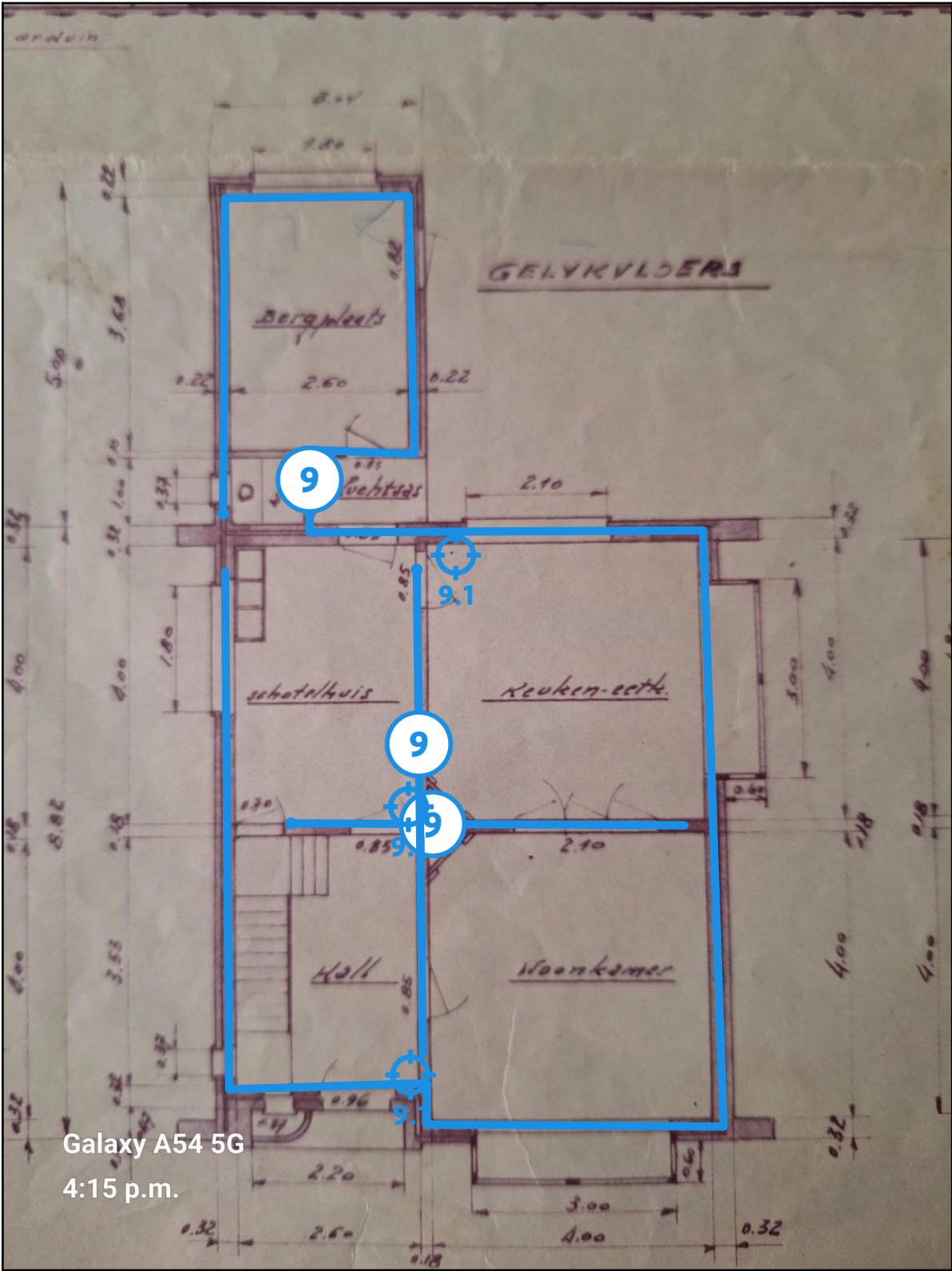
Legende van plan 1.2: Gelijkvoers - muren
