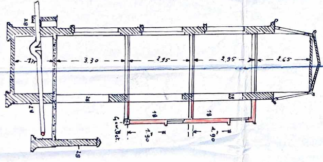
DOORSNEDE AB
