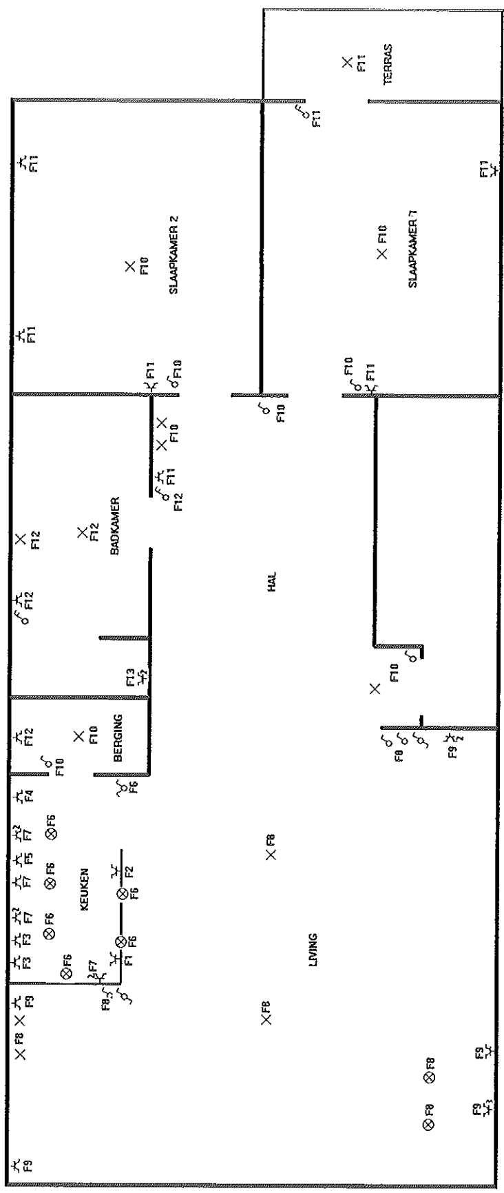
1STE VERDIEPING STOPCONTACTEN VERLICHTING SCHEMA
