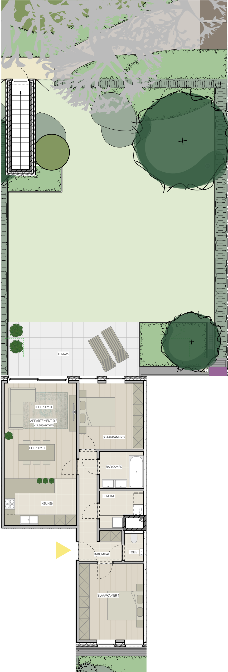
GELIJKVLOERS met tuin
