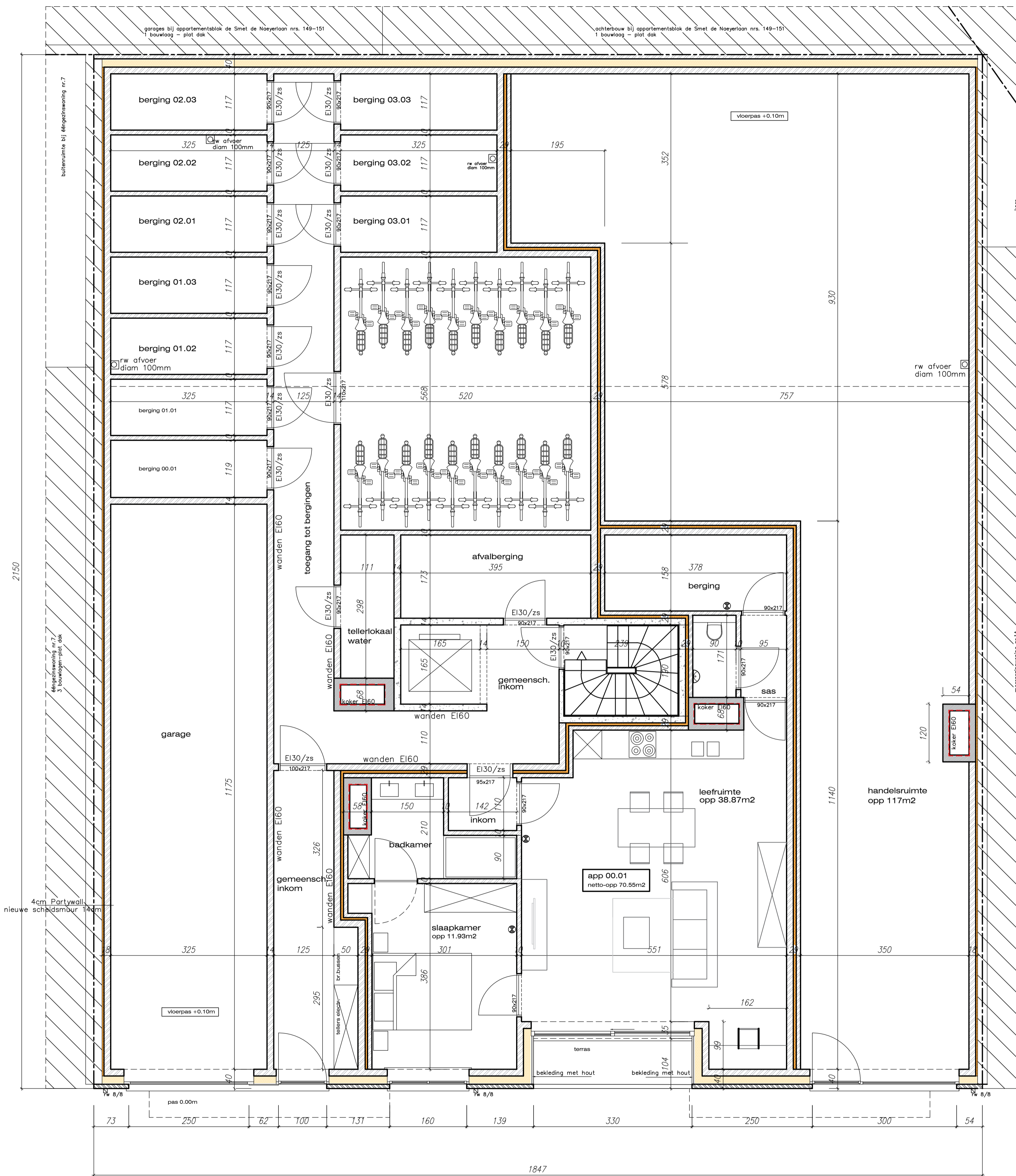
GRONDPLAN : app. 00.01- handelsruimte - garage RESIDENTIE VICTOR
