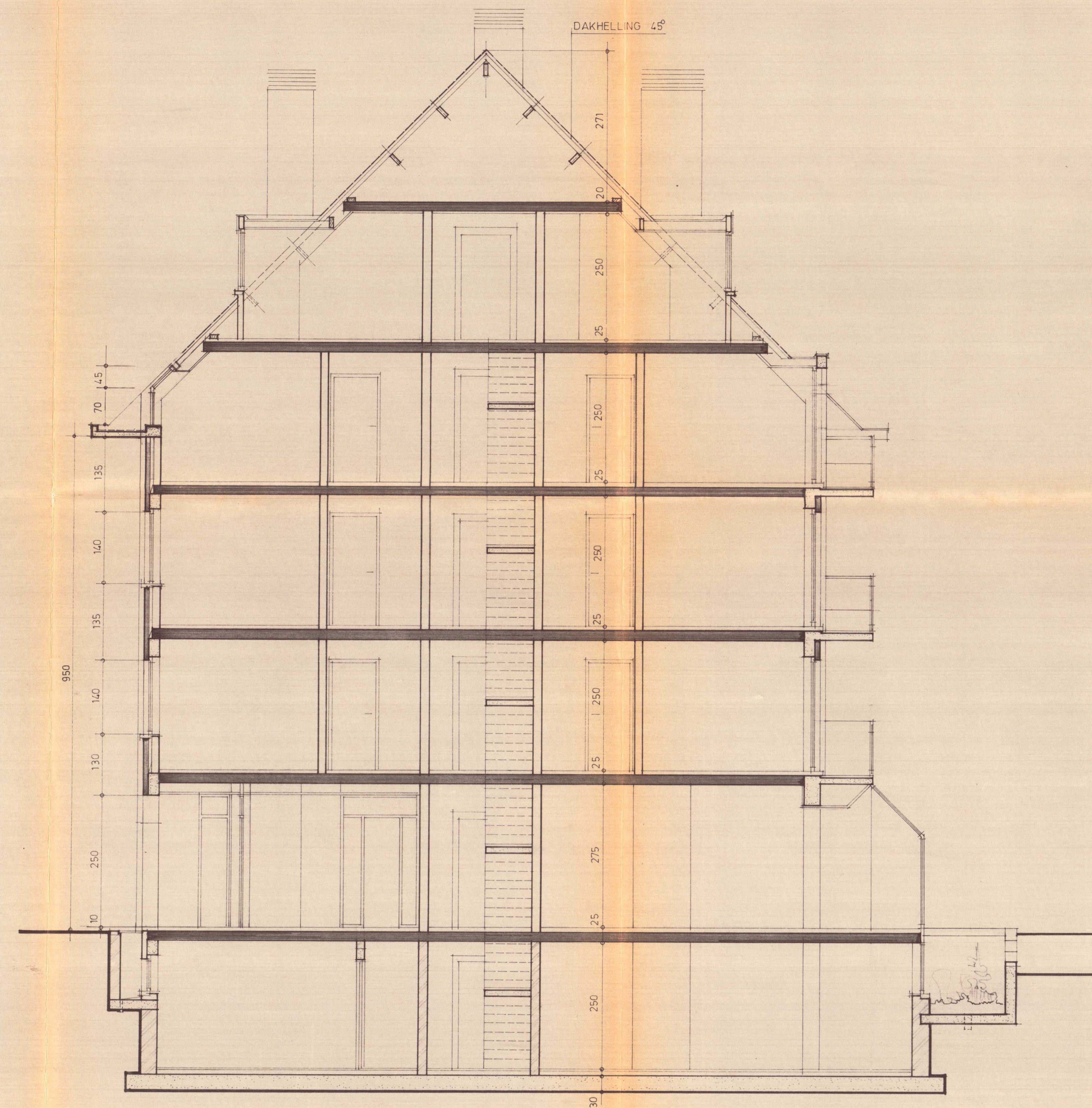
DOORSNEDE: A.B
