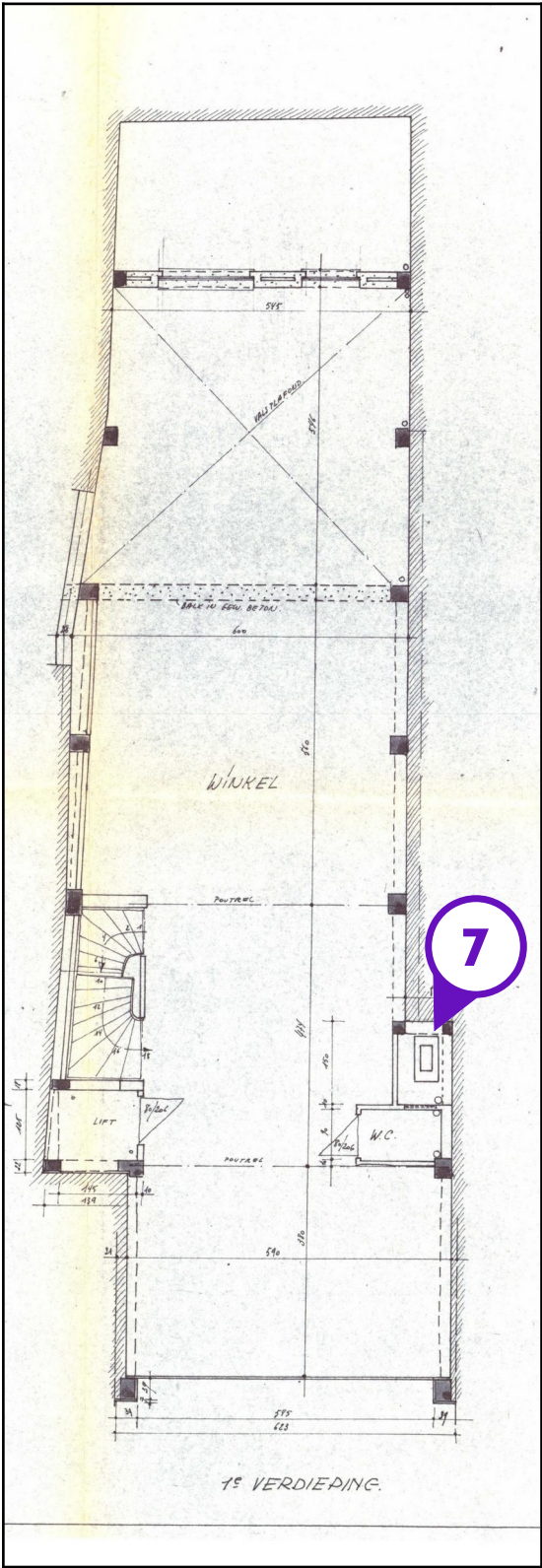
Legende van plan 1.3: Verdiep 1
