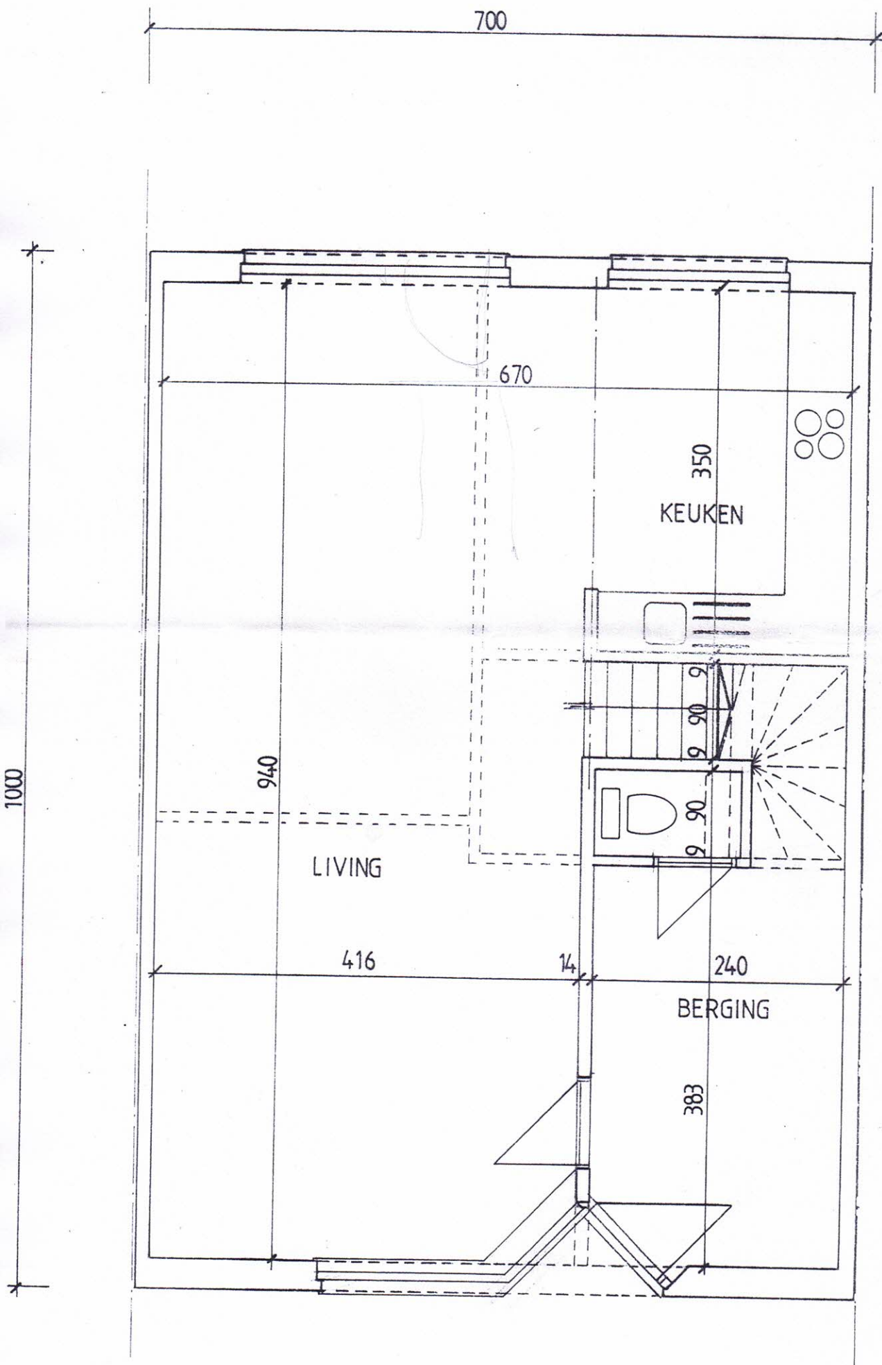
GRONDPLAN
