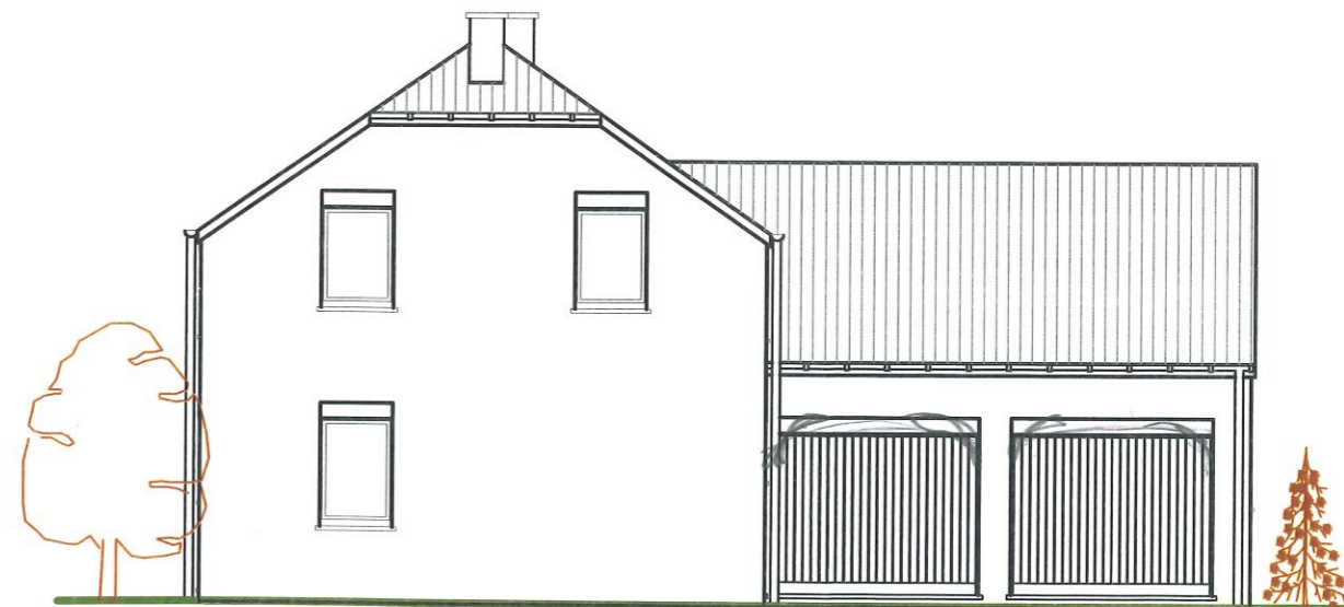
FACADE GAUCHE
