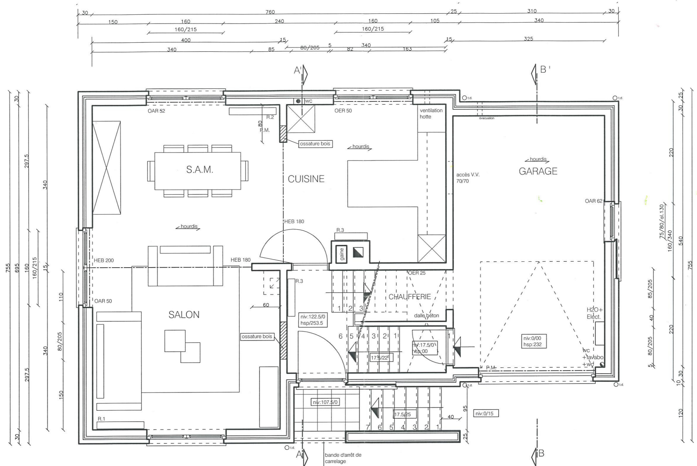
PLAN NIVEAU 0
