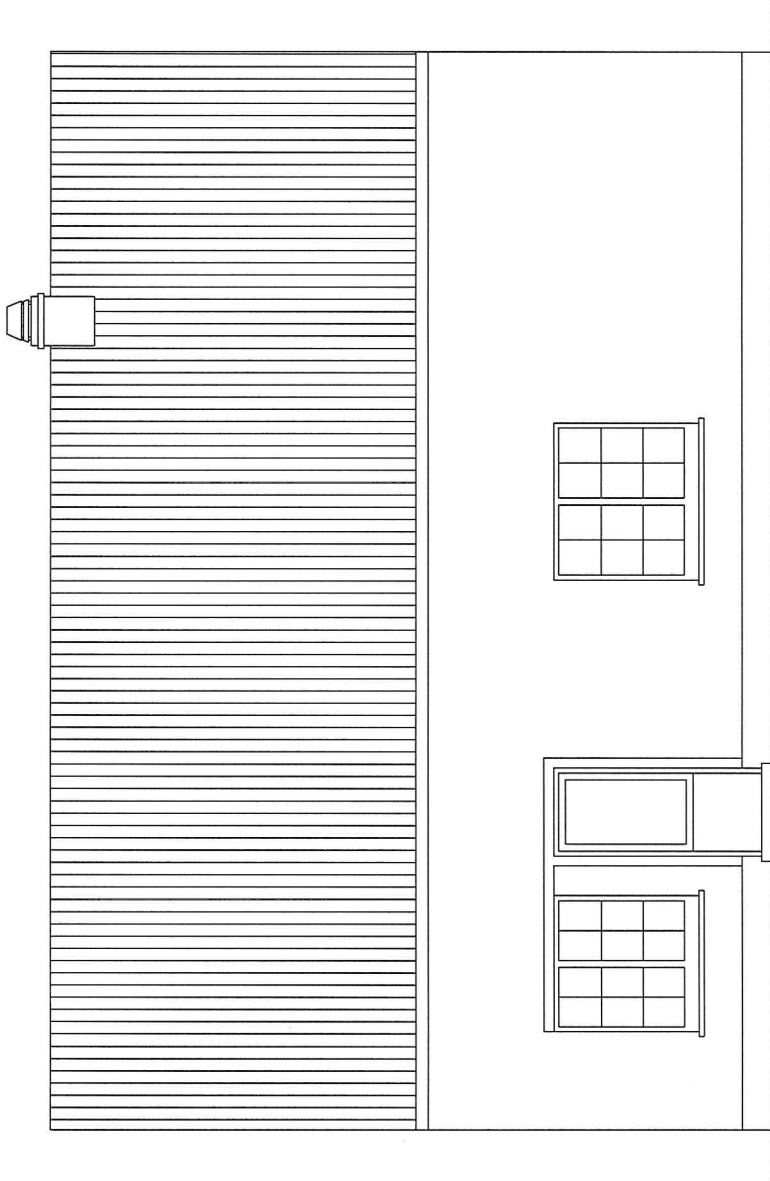
NOORDGEVEL
