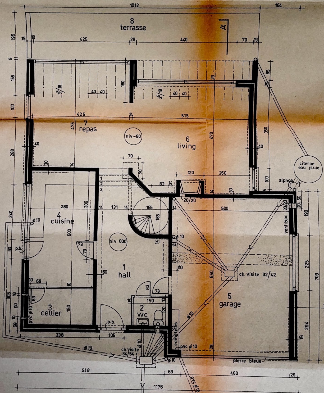
PLAN DU REZ
