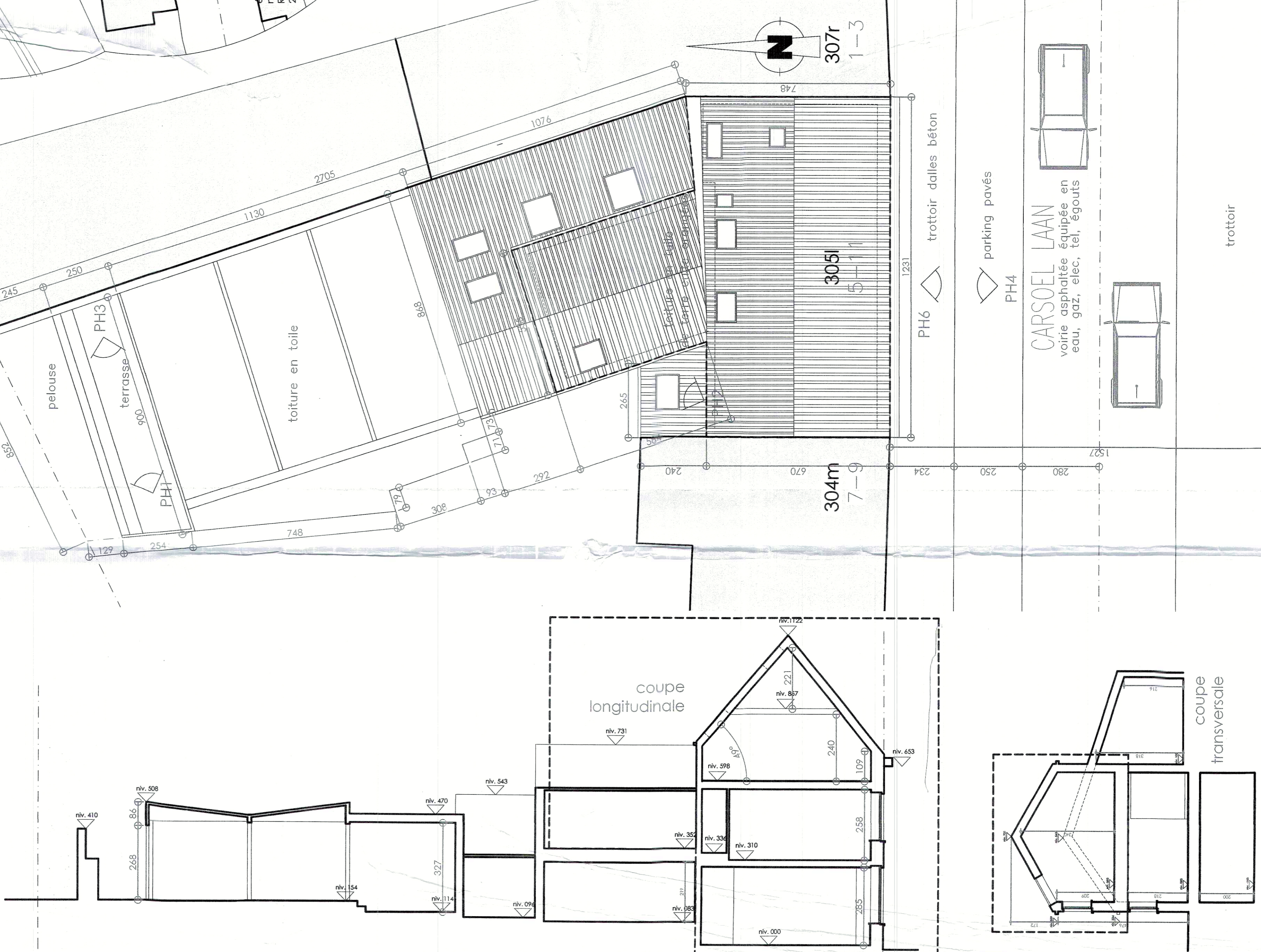
plan d'implantation 1/500
