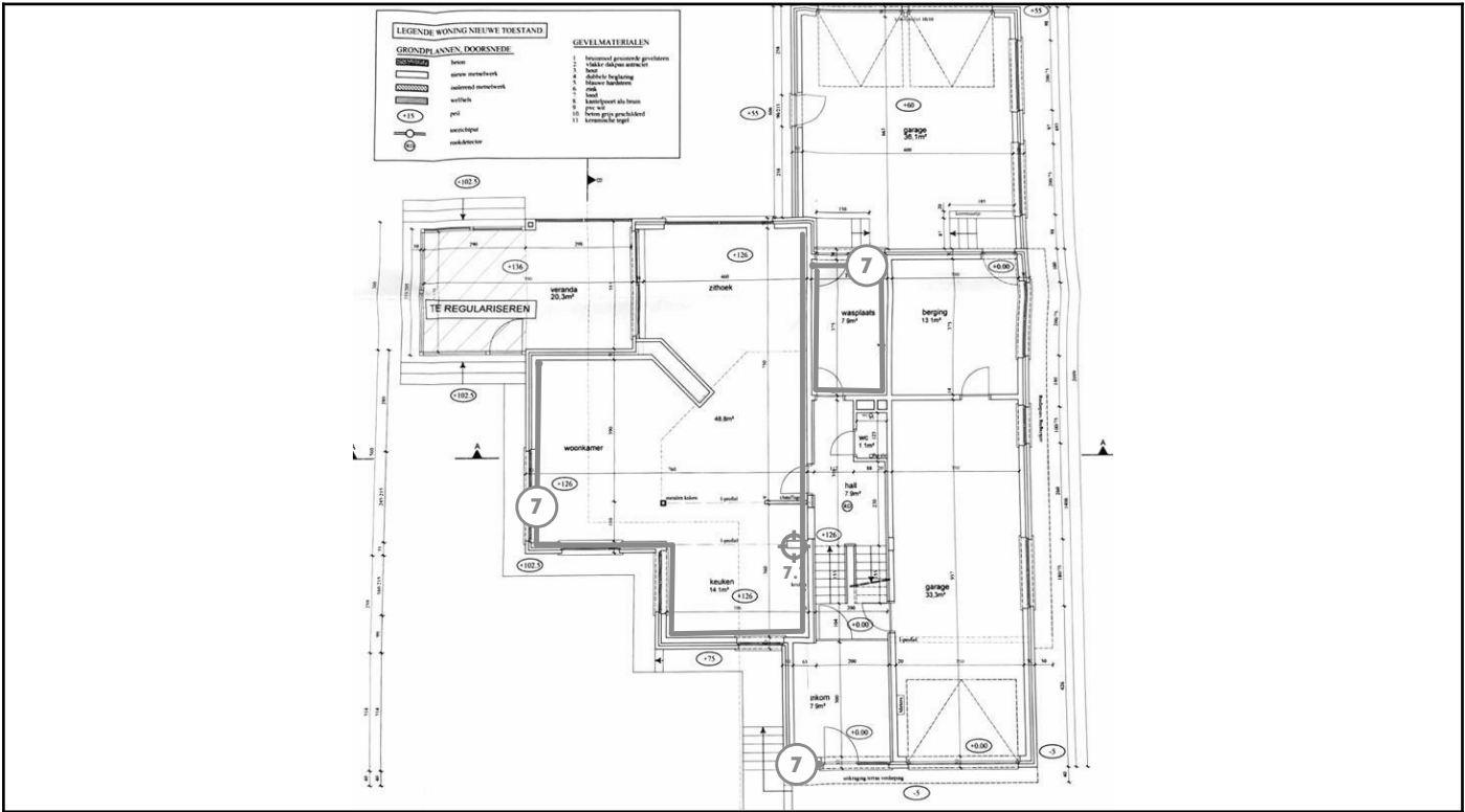
Legende van plan 1.3: gelijksvloer
