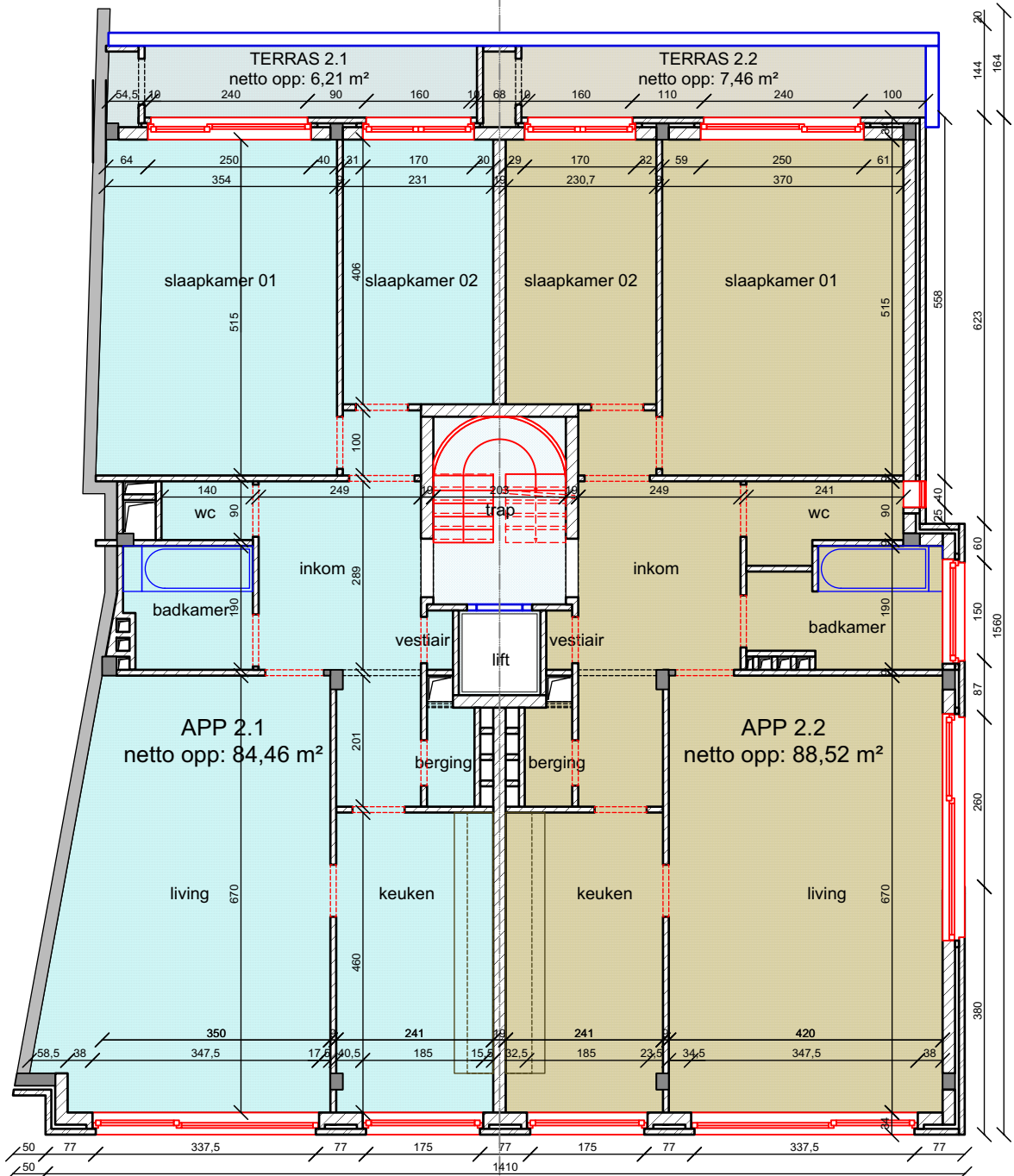
TWEDE VERDIEPING - totale netto oppervlakte excl gemeene delen :
