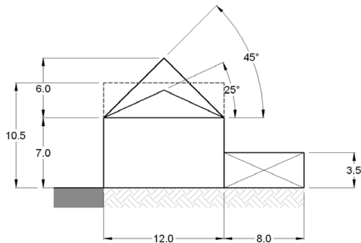
schematische voorstelling van de mogelijke bouwhoogte, -diepte en dakhelling, maximalistisch aangeduid
