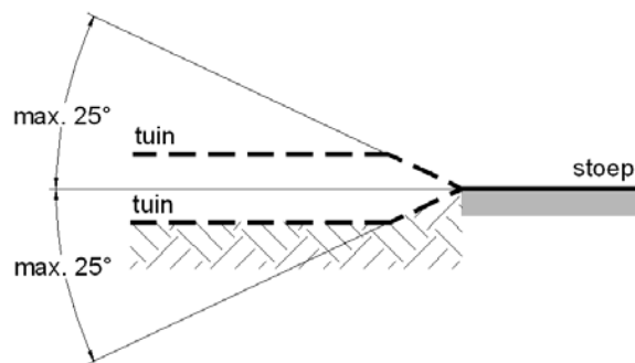
Schematische voorstelling van de maximale taludovergang tussen tuinzone en maaiveld van het voetpad.
