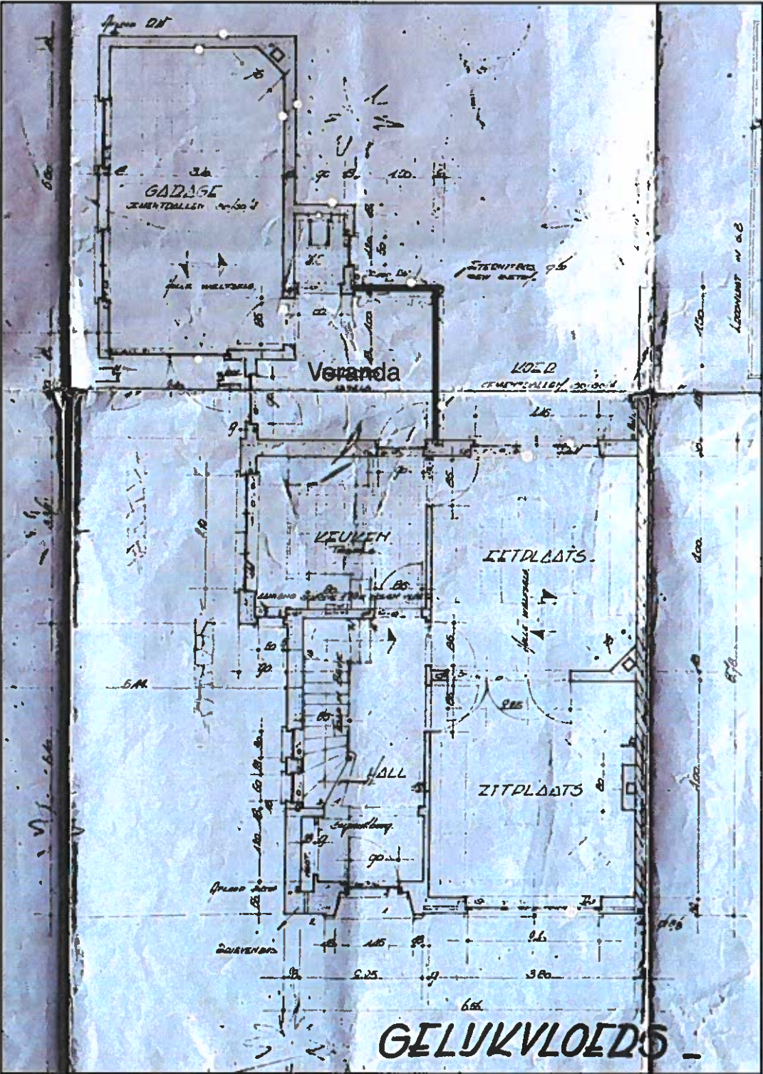
Legende van plan 1.4: Gelijkvloers
