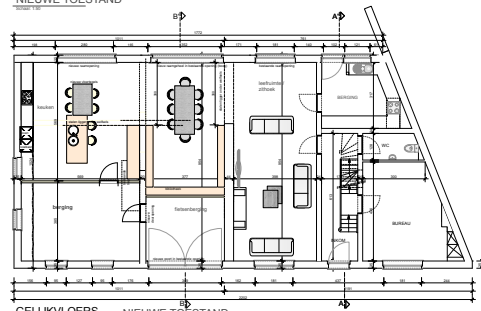
GELIJKVLOERS NIEUWE TOESTAND
