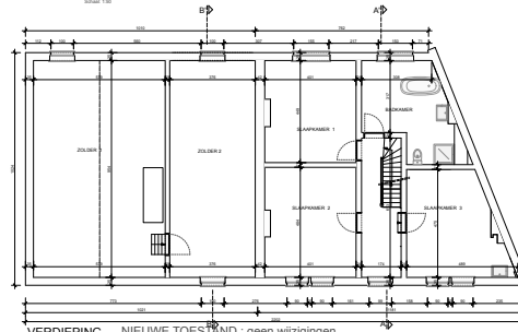
VERDIEPING NIEUWE TOESTAND : geen wijzigingen
