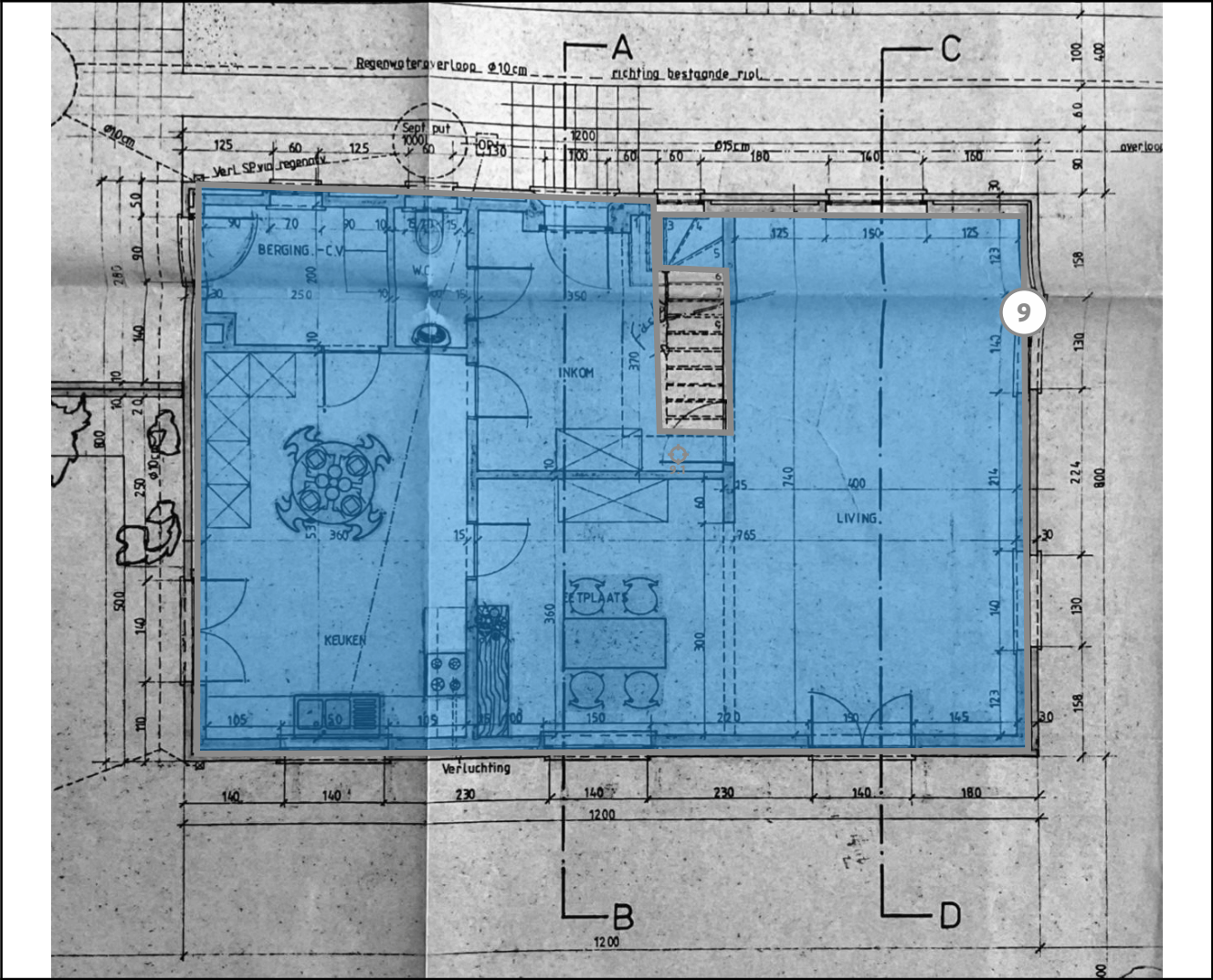
Legende van plan 1.3: Gelijkvloers
