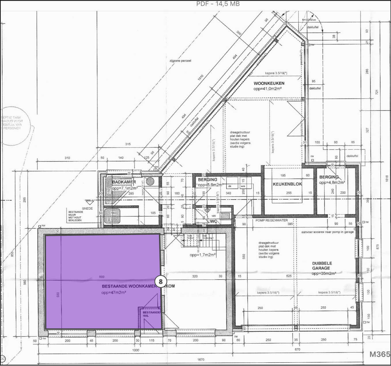
Legende van plan 1.3: Gelijkvloers
